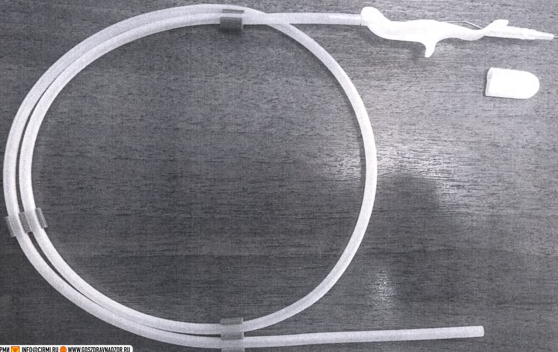
Фото 12. Проводник Lunderquist
