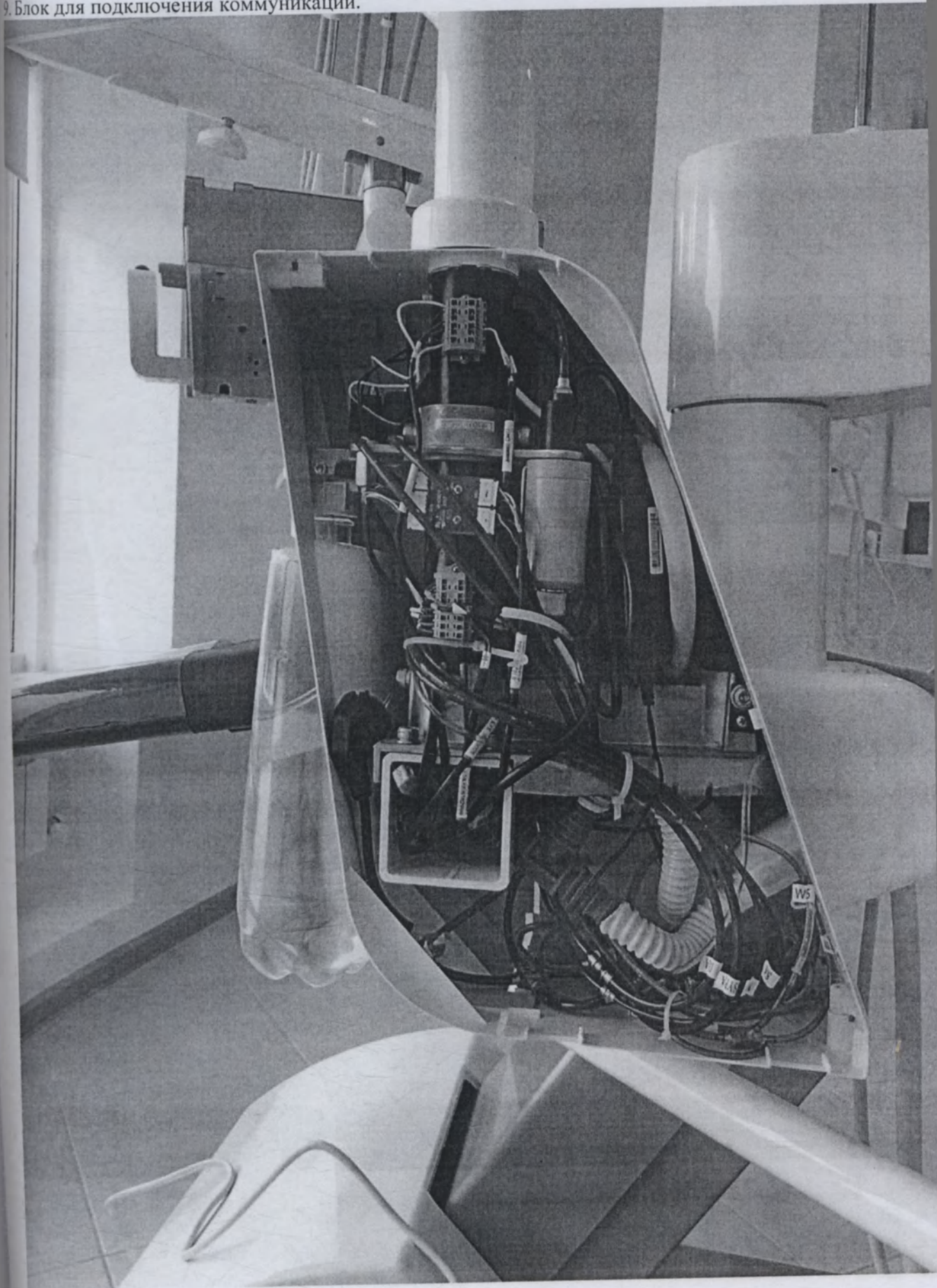
9. Блок для подключения коммуникаций.
