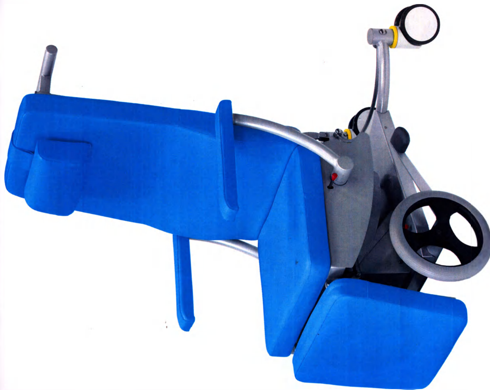
Кресло медицинское многофункциональное передвижное КММП-03
