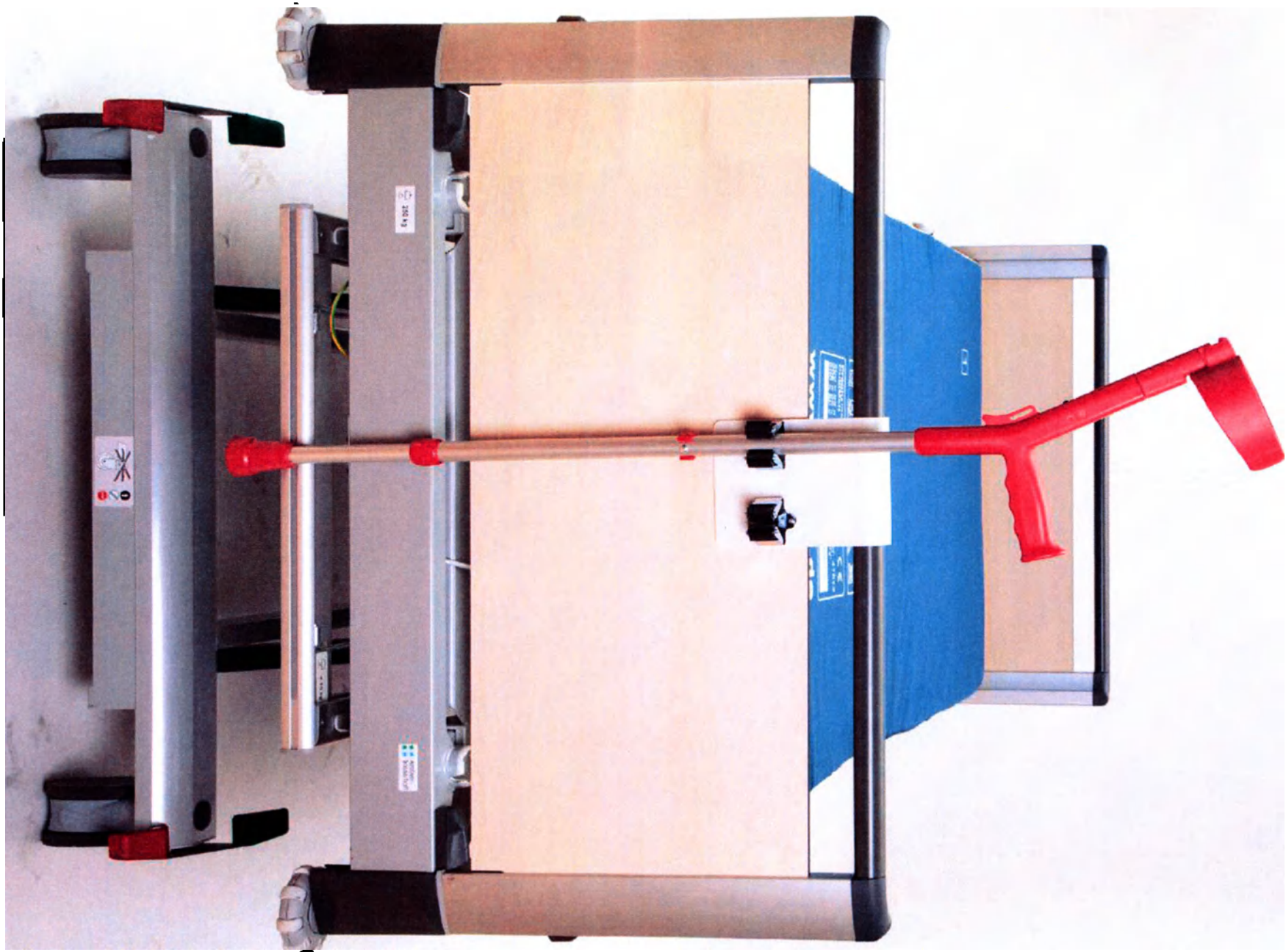
Держатель для костылей с креплением на торцевое ограждение
