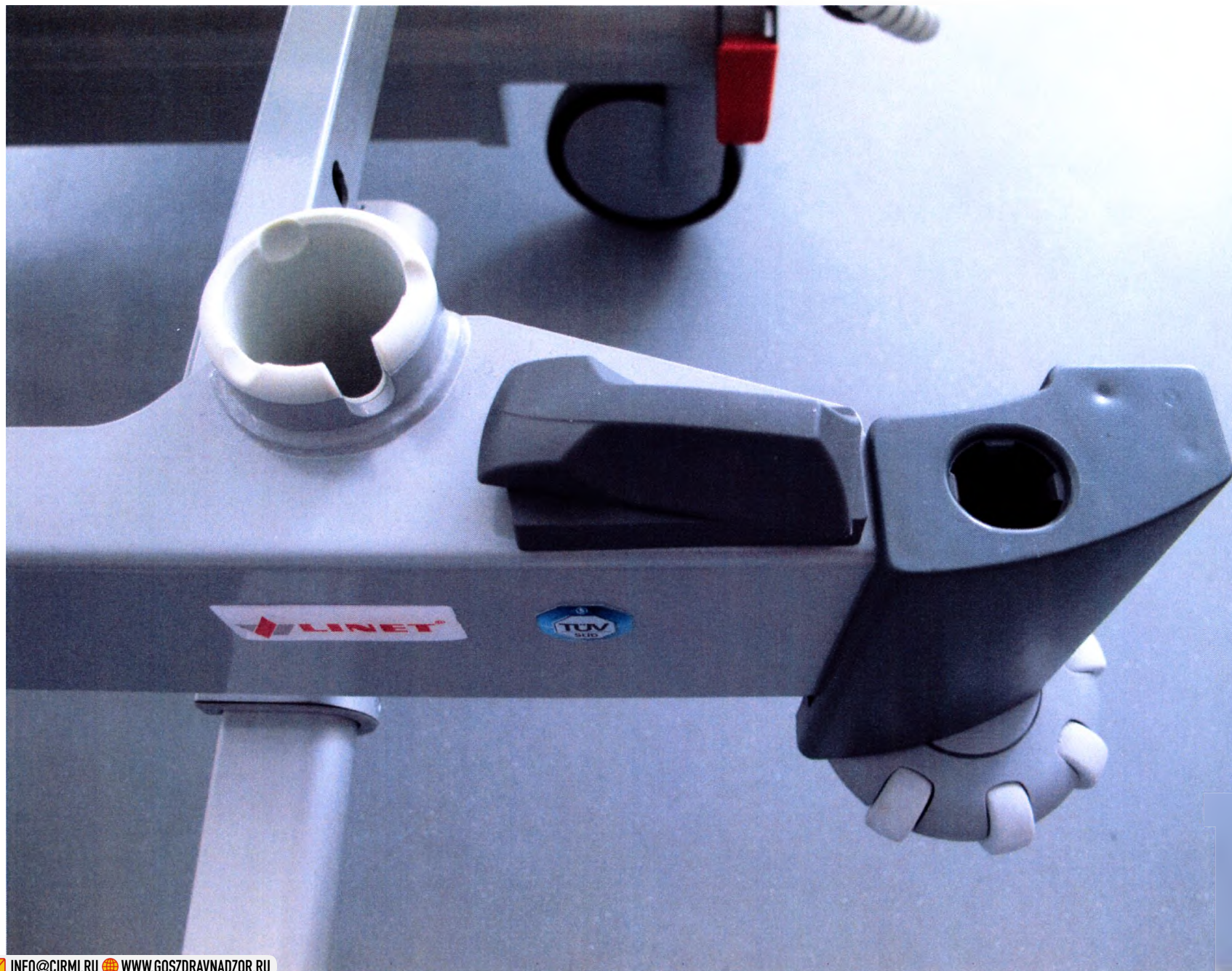
Механизм фиксации торцевых ограждений, интегрированный в раму матрасной платформы
