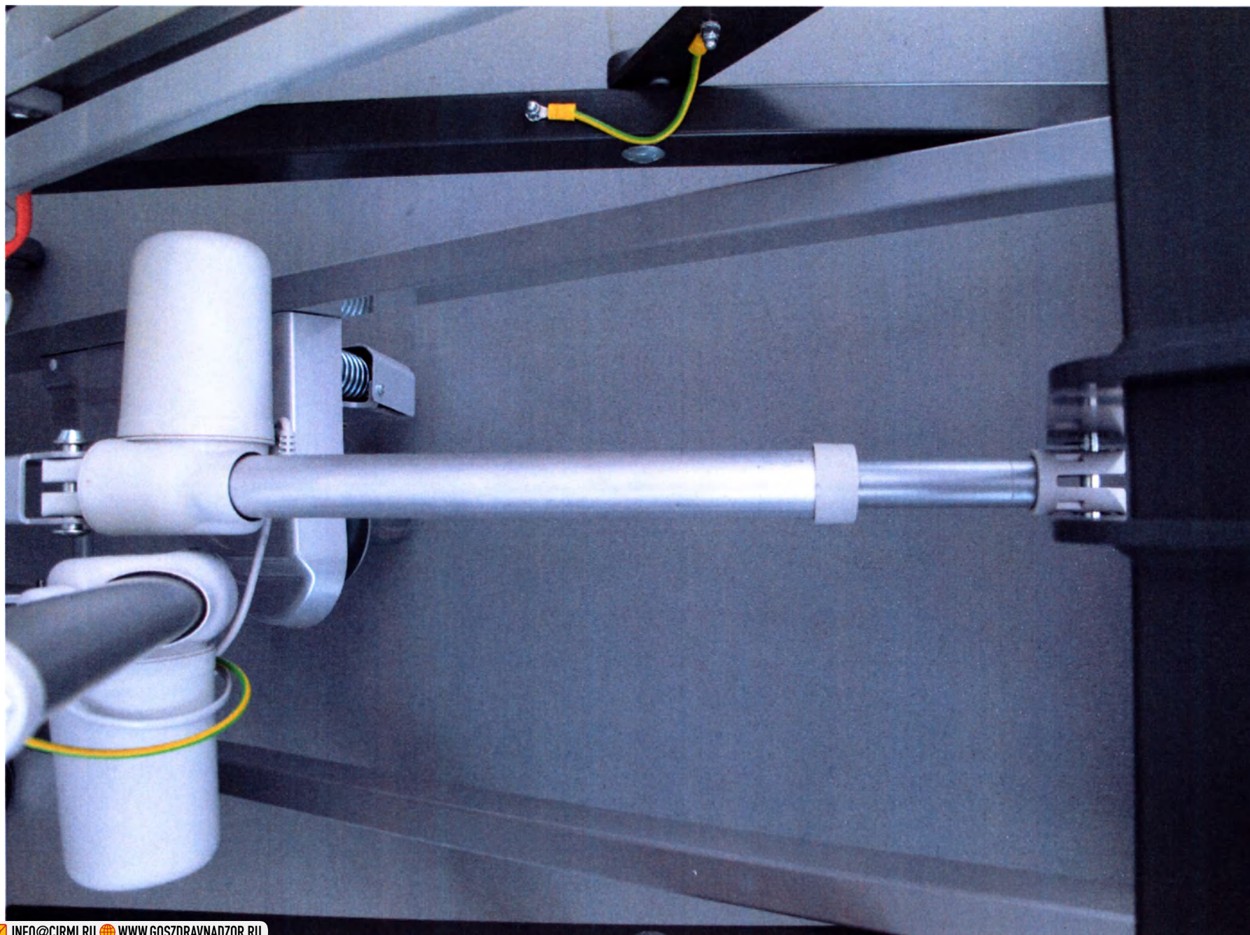
Двигатель линейный с приводом регулировки высоты и наклона ложа
