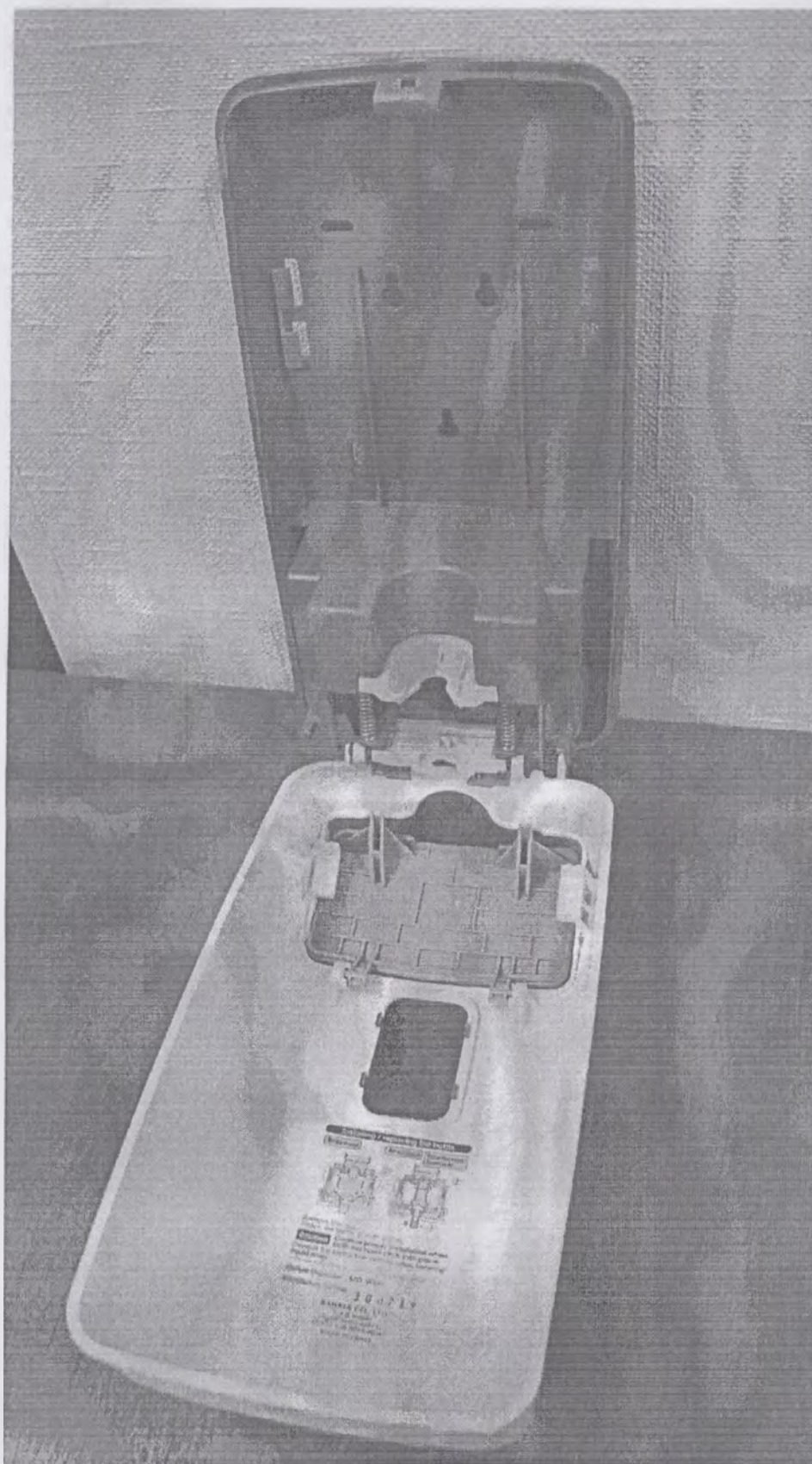
ФОТО 3. МЕХАНИЧЕСКИЙ ДОЗАТОР SARAYA МОДЕЛИ MD-9000 В ОТКРЫТОМ ВИДЕ
