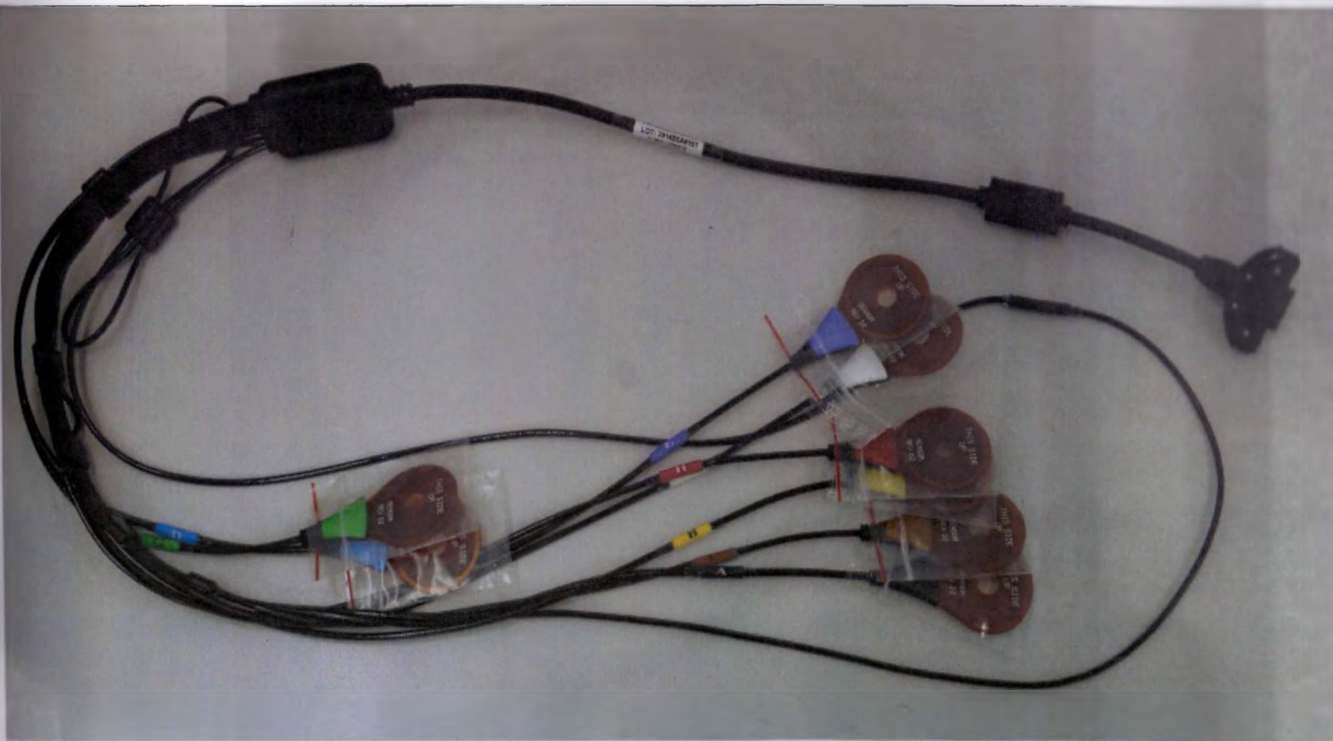
13. Датчики SensorArray с 8-ю проводами и кабелем подключения к регистрирующему устройству
