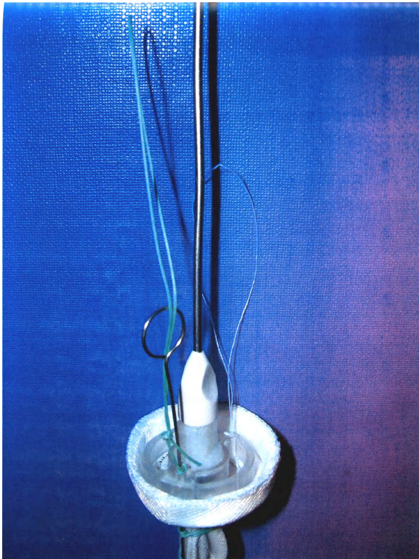
Стент-графт, закреплённый на системе доставки
