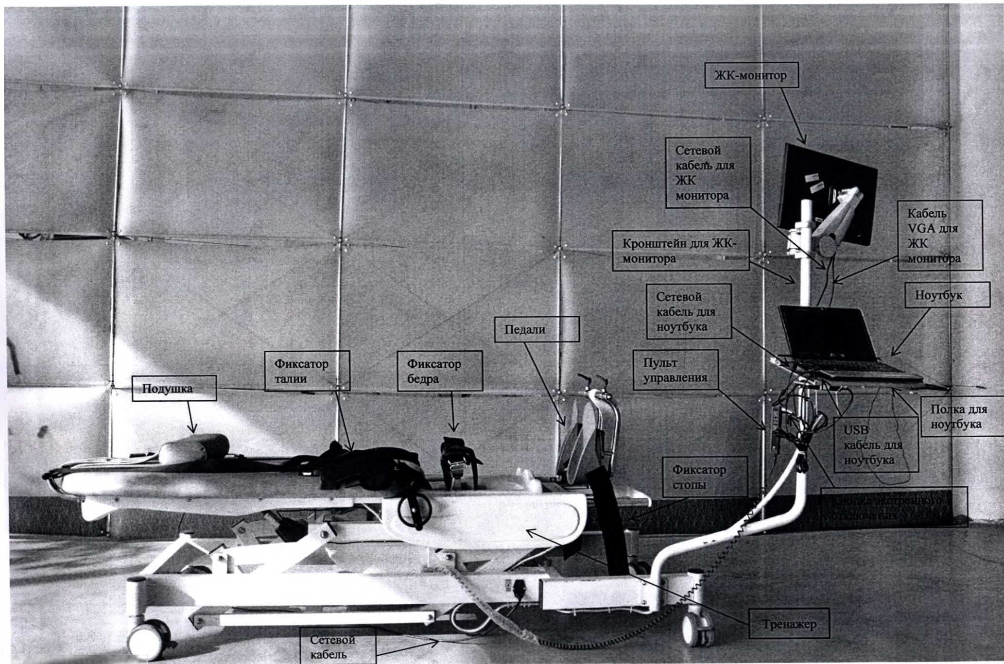
Интеллектуальная система тренировки с биологической обратной связью для нижних конечностей А1
