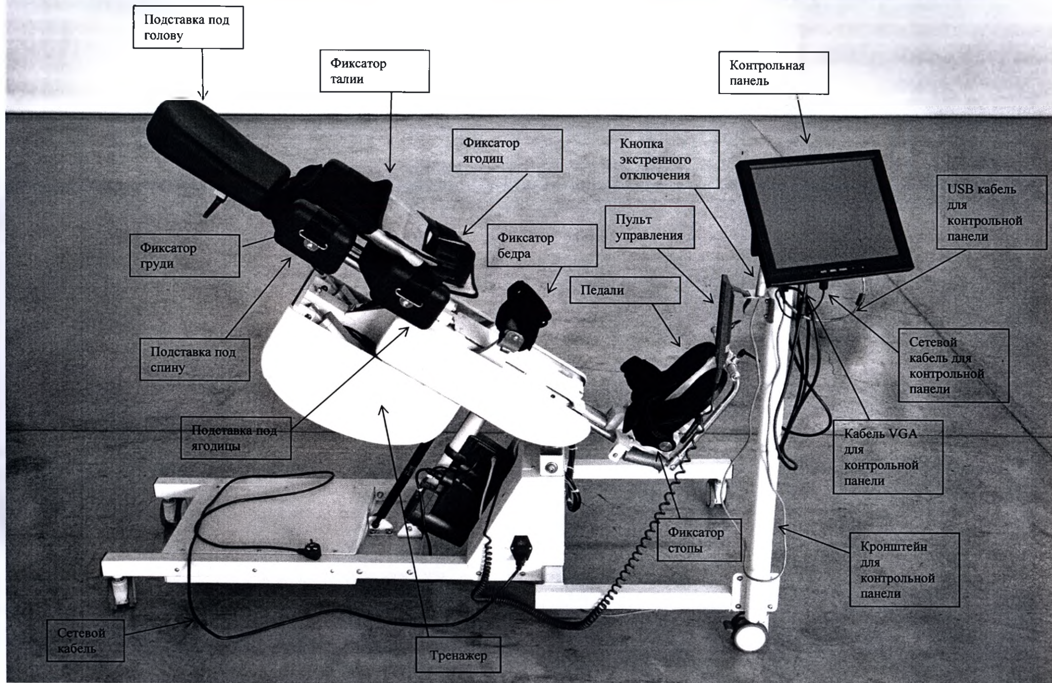
Интеллектуальная система тренировки с биологической обратной связью для нижних конечностей С1
