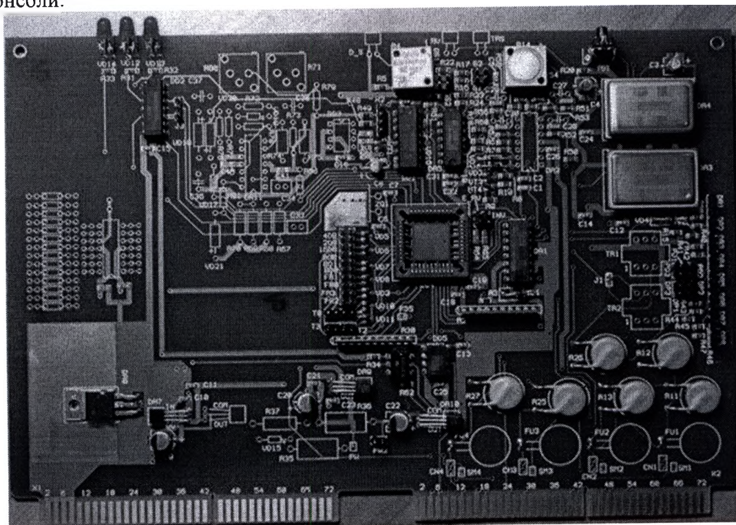
29. Плата консоли.
