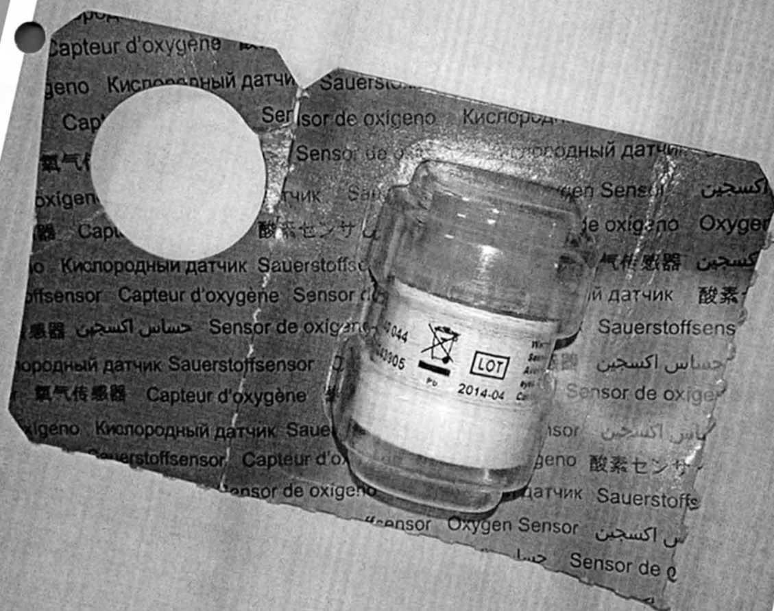
ЯЧЕЙКА КИСЛОРОДНАЯ
