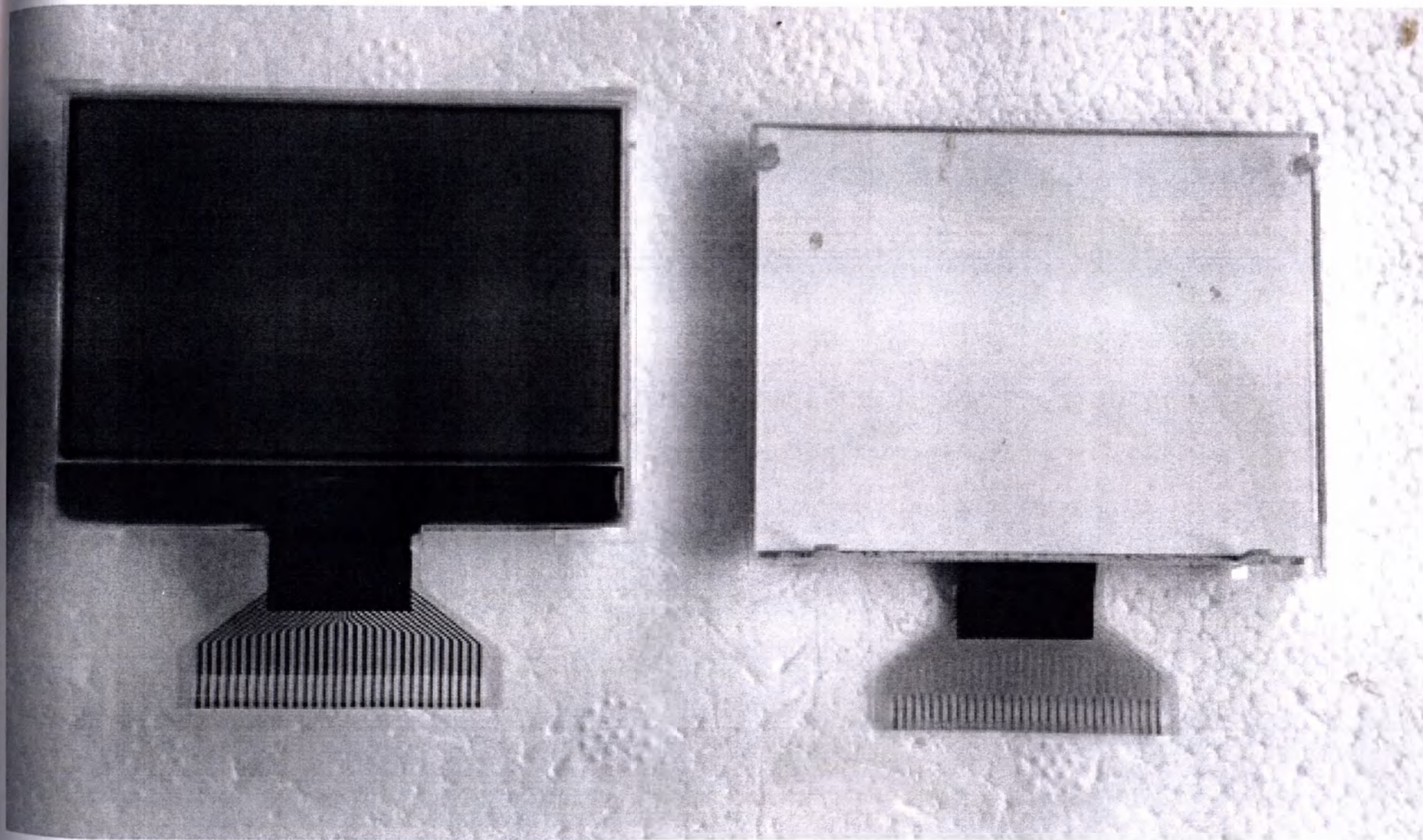
Дисплей (FSTN) с соединительным кабелем
