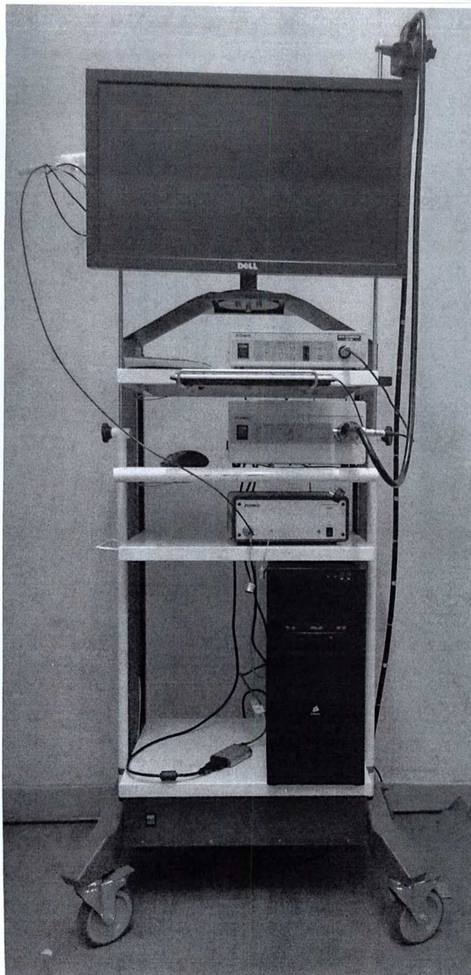
Эндовидеосистема для исследования желудочно-кишечного тракта методом оптической когерентной томографии ЭВС-ОКТ
