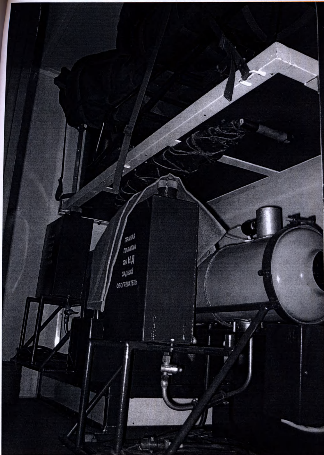
Фотография 8. Автоперевязочная АП-2-«СЗМО» в кузове-фургоне К4310 на шасси автомобиля КАМАЗ 43114 по ТУ 9451-004-07614018-2008. Грузовое отделение с правой стороны
