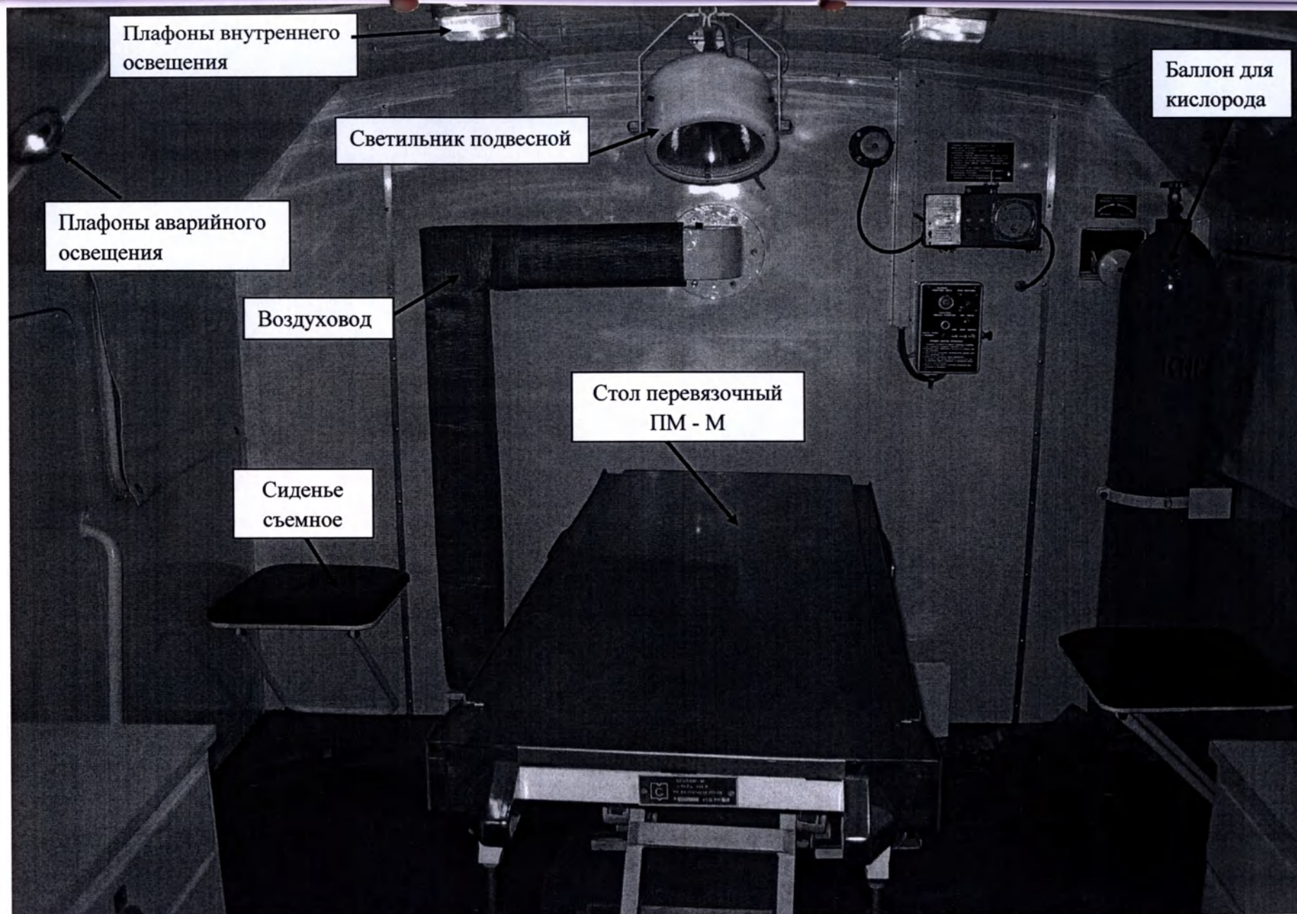
Фотография 5. Автоперевязочная АП-2-«СЗМО» в кузове-фургоне К4310 на шасси автомобиля КАМАЗ 43114 по ТУ 9451-004-07614018-2008. Перевязочное отделение внутри кузова-фургона. Общий вид.
