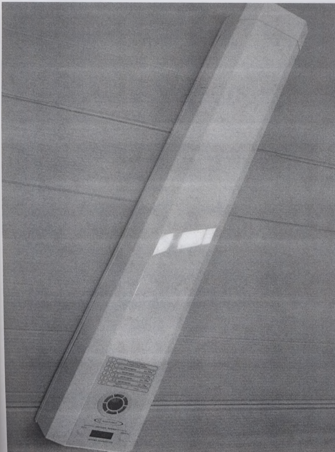
Фотография 2. Медицинское изделие «Рециркулятор УФ-бактерицидный двухламповый с принудительной циркуляцией воздушного потока для обеззараживания воздуха помещений в присутствии людей РБ-06-«Я-ФП» по ТУ 9451-006-55307168-2004. Исполнение РБ-06-«Я-ФП»-01. Общий вид.
