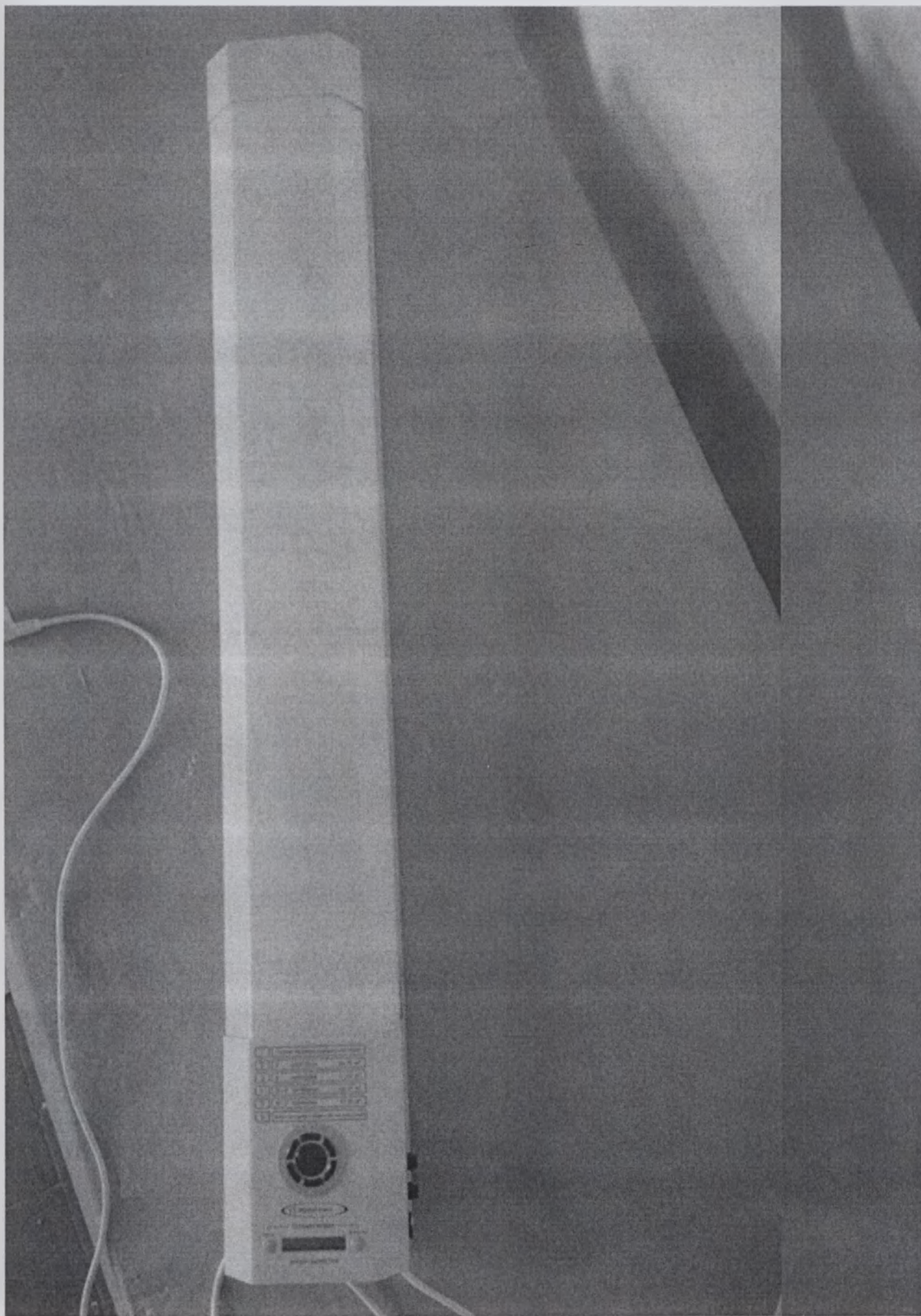
Фотография 8. Медицинское изделие «Рециркулятор УФ-бактерицидный двухламповый с принудительной циркуляцией воздушного потока для обеззараживания воздуха помещений в присутствии людей РБ-06-«Я-ФП» по ТУ 9451-006-55307168-2004. Исполнение РБ-06-«Я-ФП»-02. Общий вид.
