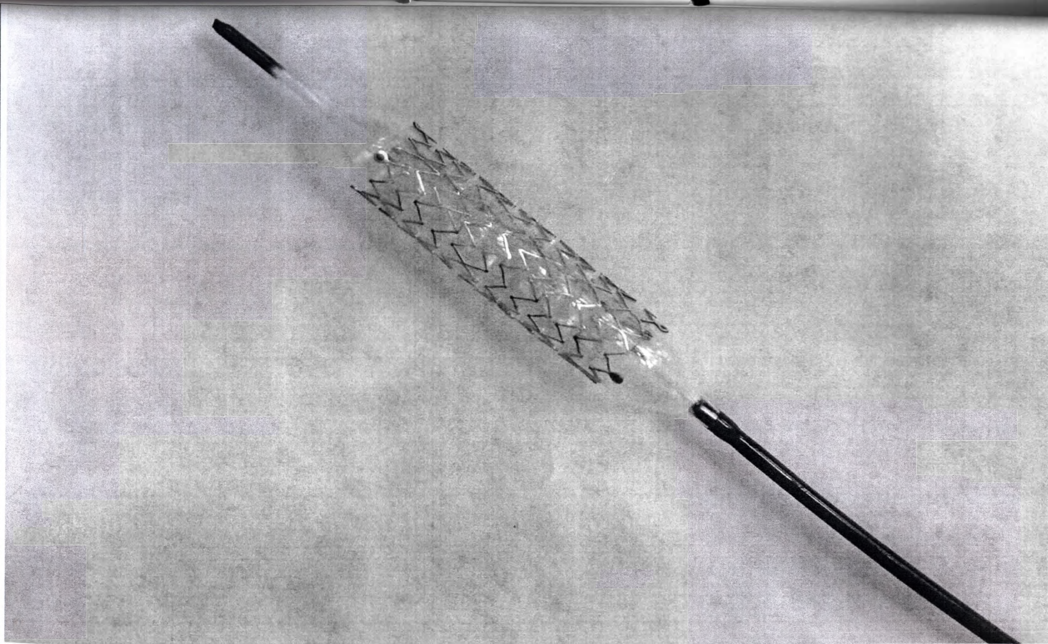
Система для стентирования периферических сосудов ParaMount Mini GPS с баллонорасширяемым стентом (стент предустановленный на баллонном катетере)
