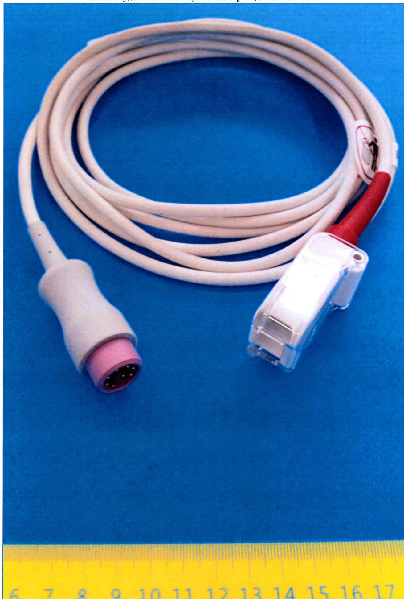
Кабель удлинительный, Masimo SpO2, 8-контактный
