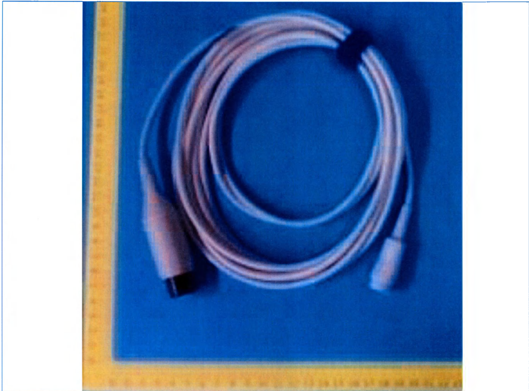
Кабель инвазивного давления, 6-контактный
