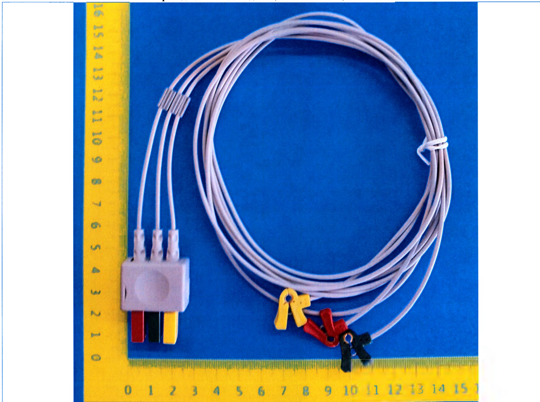
Провод ЭКГ на 3 отведения, неонатальный, тип зажим
