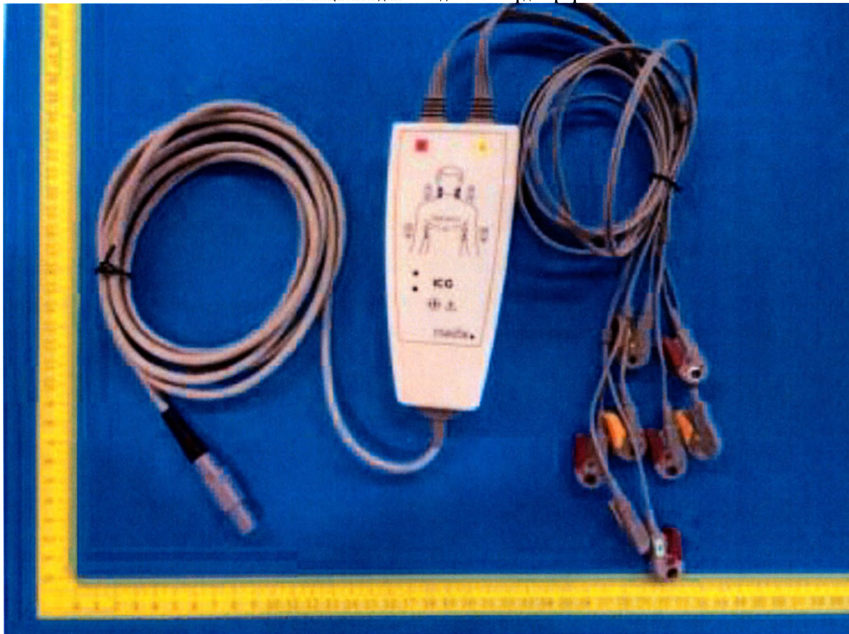
Кабель пациента для импедансной кардиографии
