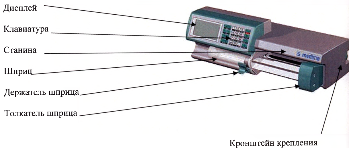
Рис. 2. Модель S-PCA
