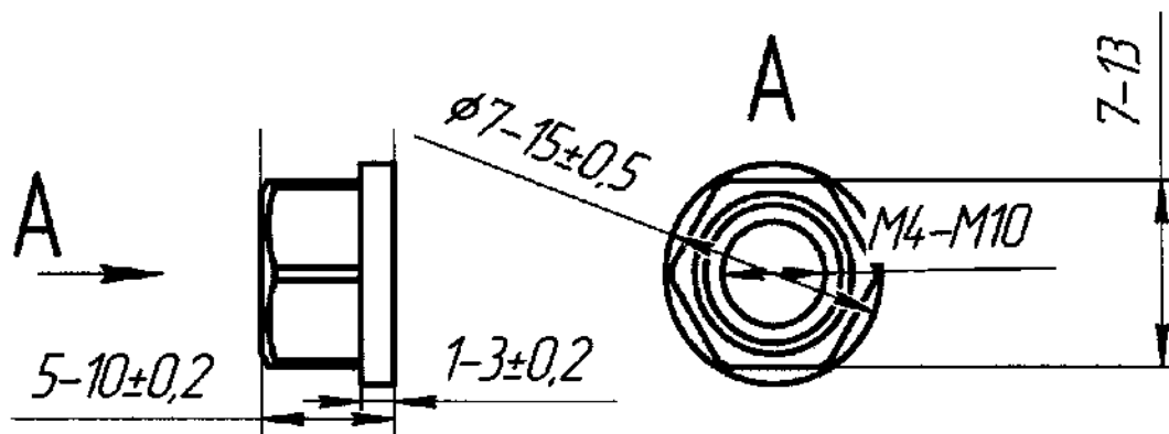
А.10 - Гайка
