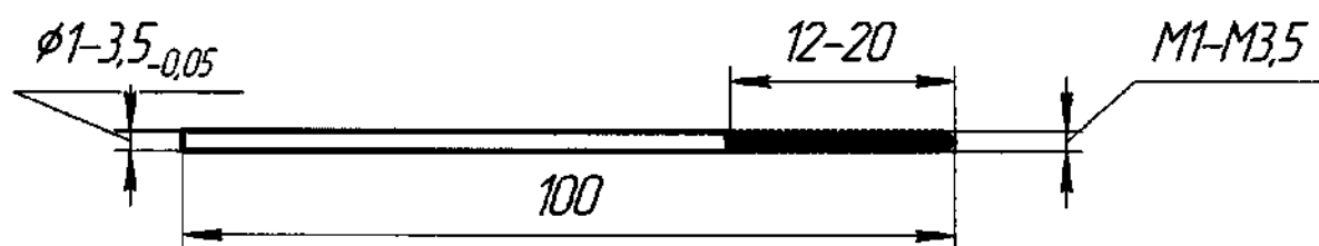
Рисунок А.12 – Спица Киршнера
