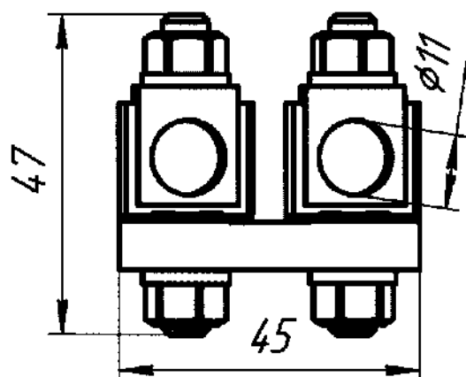
Рисунок А.2 – Зажим двойной параллельный
