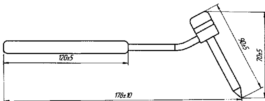
Рисунок А.14 – Направитель
