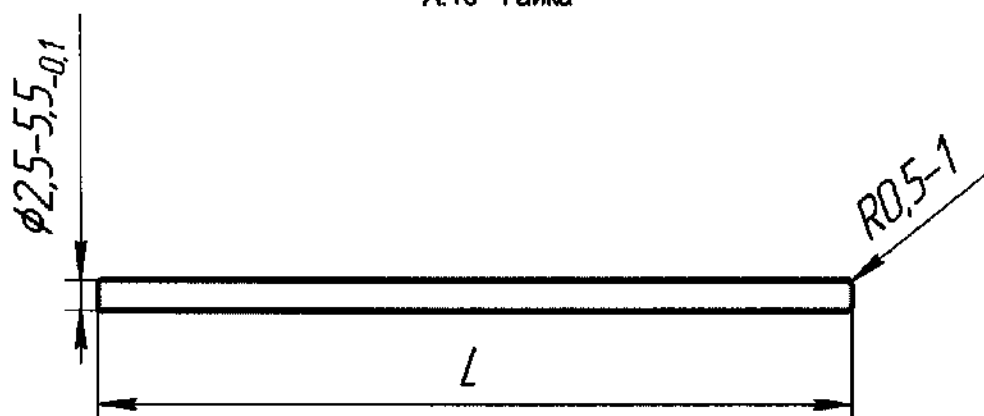
Рисунок А.11 – Штанга несущая
