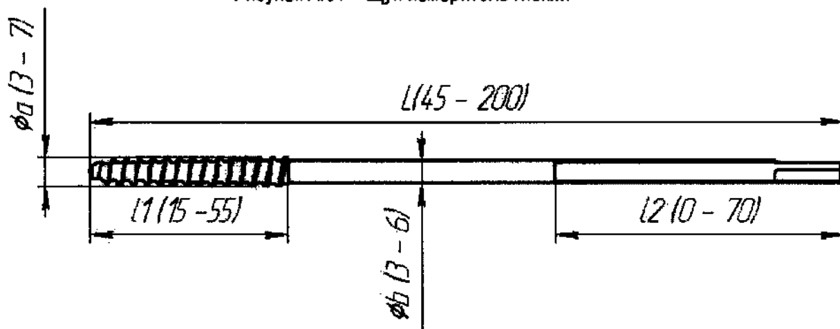
Рисунок А.31 – Щуп измеритель гибкий
