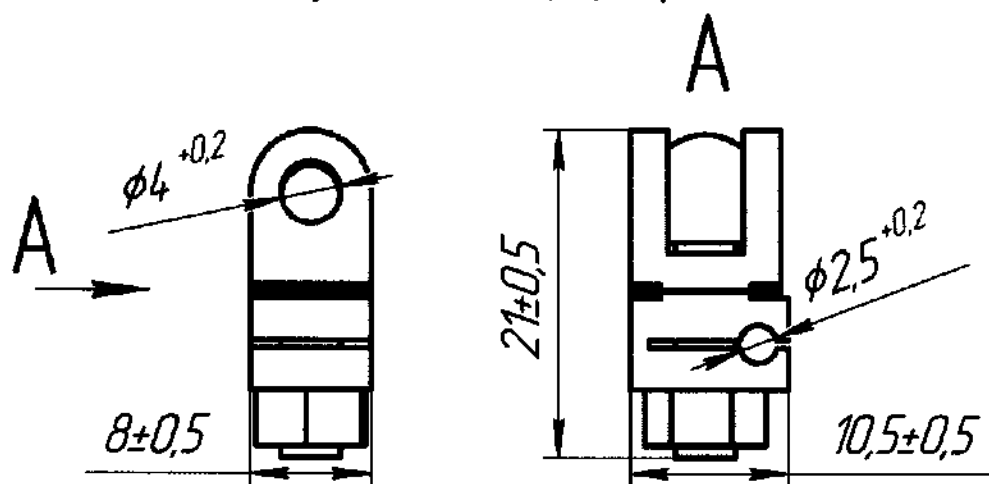
Рисунок А.7 – Зажим 4,0/2,5 закрытый
