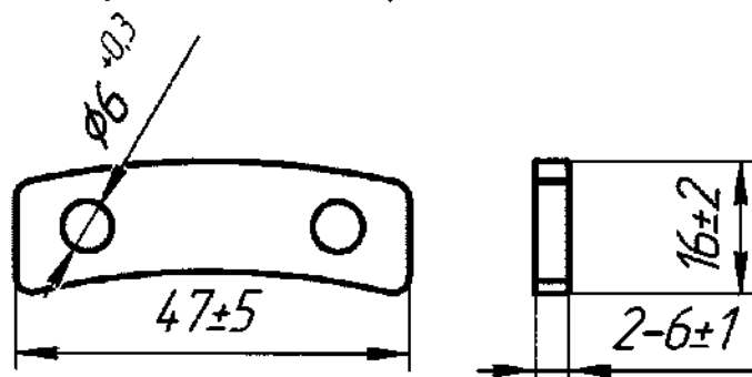
Рисунок А. 38 – Блок фиксации спиц
