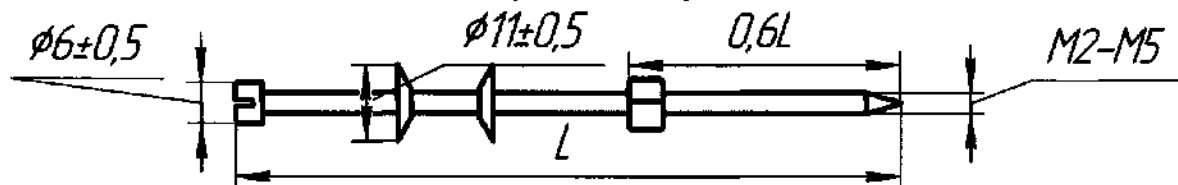
Рисунок А.16 – Болт – стяжка
