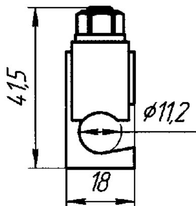
Рисунок А.1 – Зажим открытый
