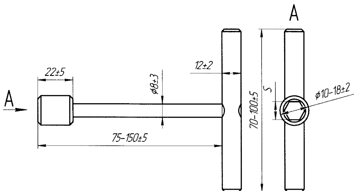
Рисунок А.28 – Ключ торцевой
