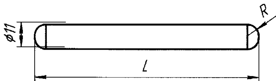
Рисунок А.5 – Трубка несущая
