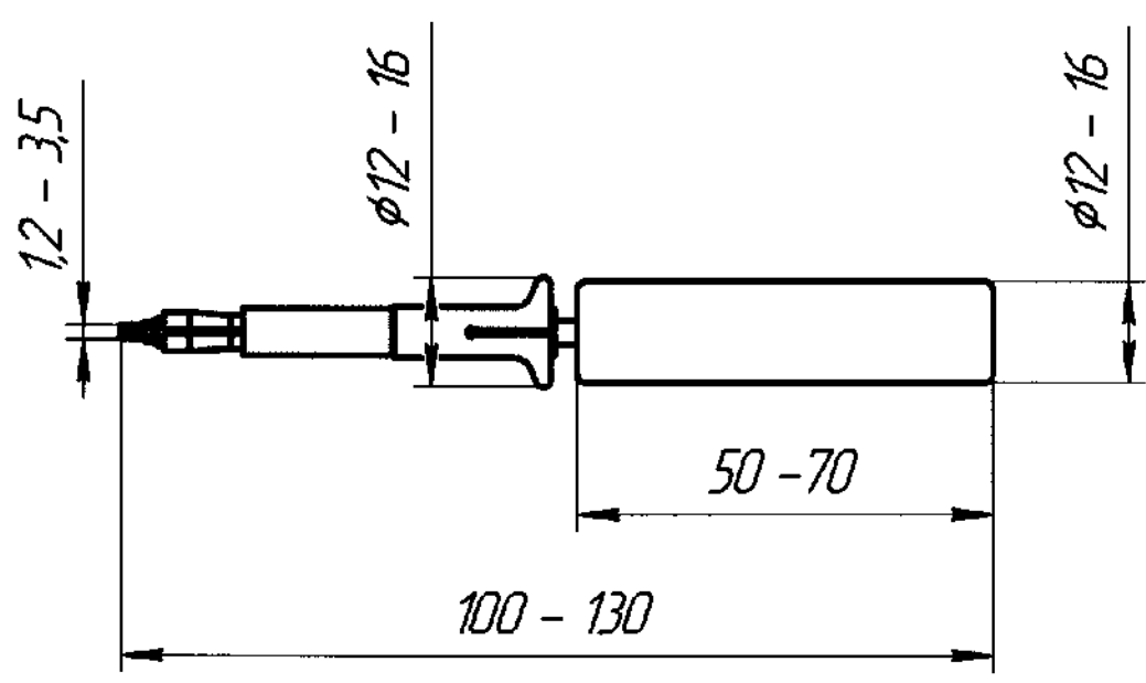
Рисунок А. 35 – Отвертка цанговая
