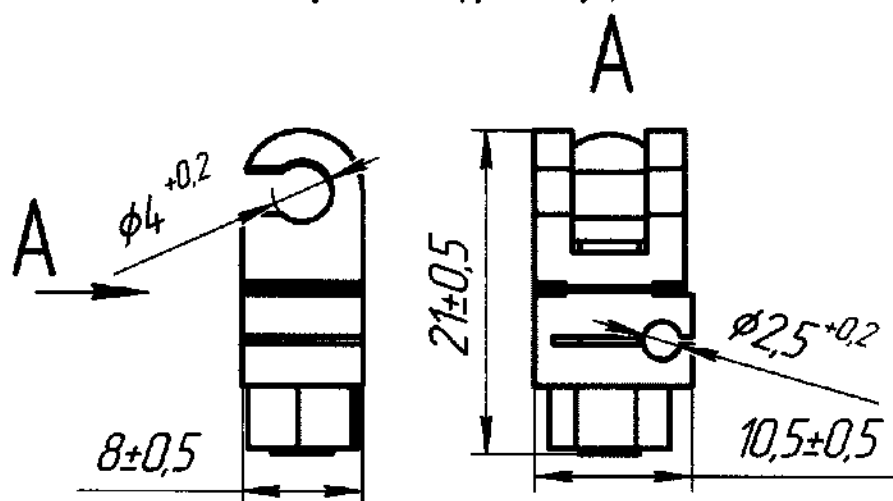
Рисунок А.6 – Зажим 4,0/2,5 открытый
