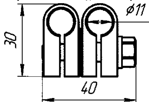
Рисунок А.3 – Зажим «трубка к трубке»
