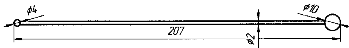
Рисунок А.31 – Щуп измеритель гибкий
