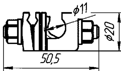
Рисунок А.4 – Зажим универсальный
