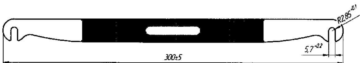
Рисунок А.23 – Ключ изгибающий
