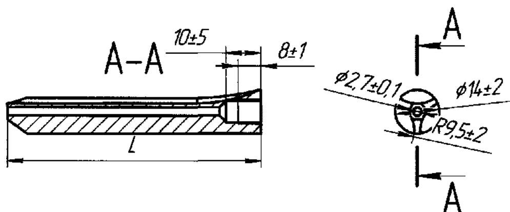
Рисунок А.17 – Гвоздь трехгранный
