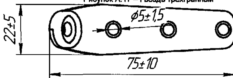
Рисунок А.18 – Накладка гвоздя трехгранного
