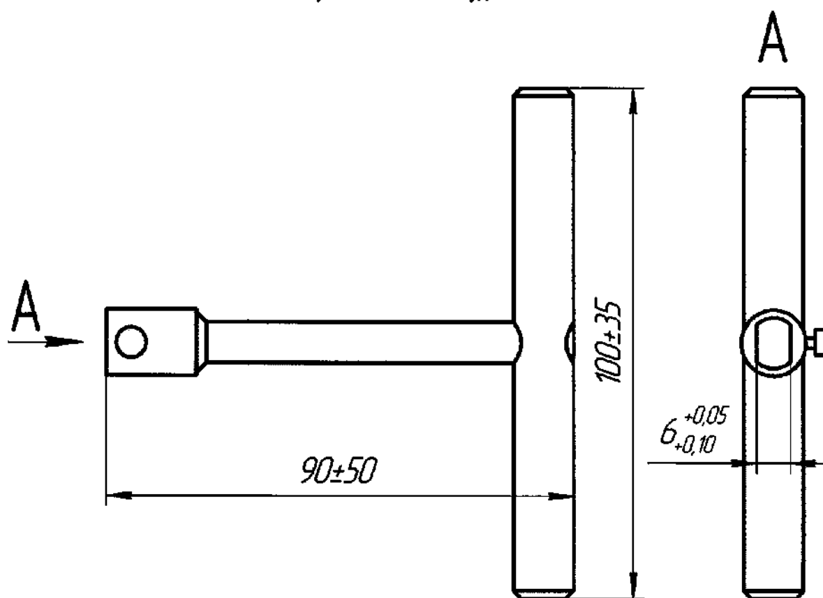
Рисунок А.25 – Ключ удерживающий
