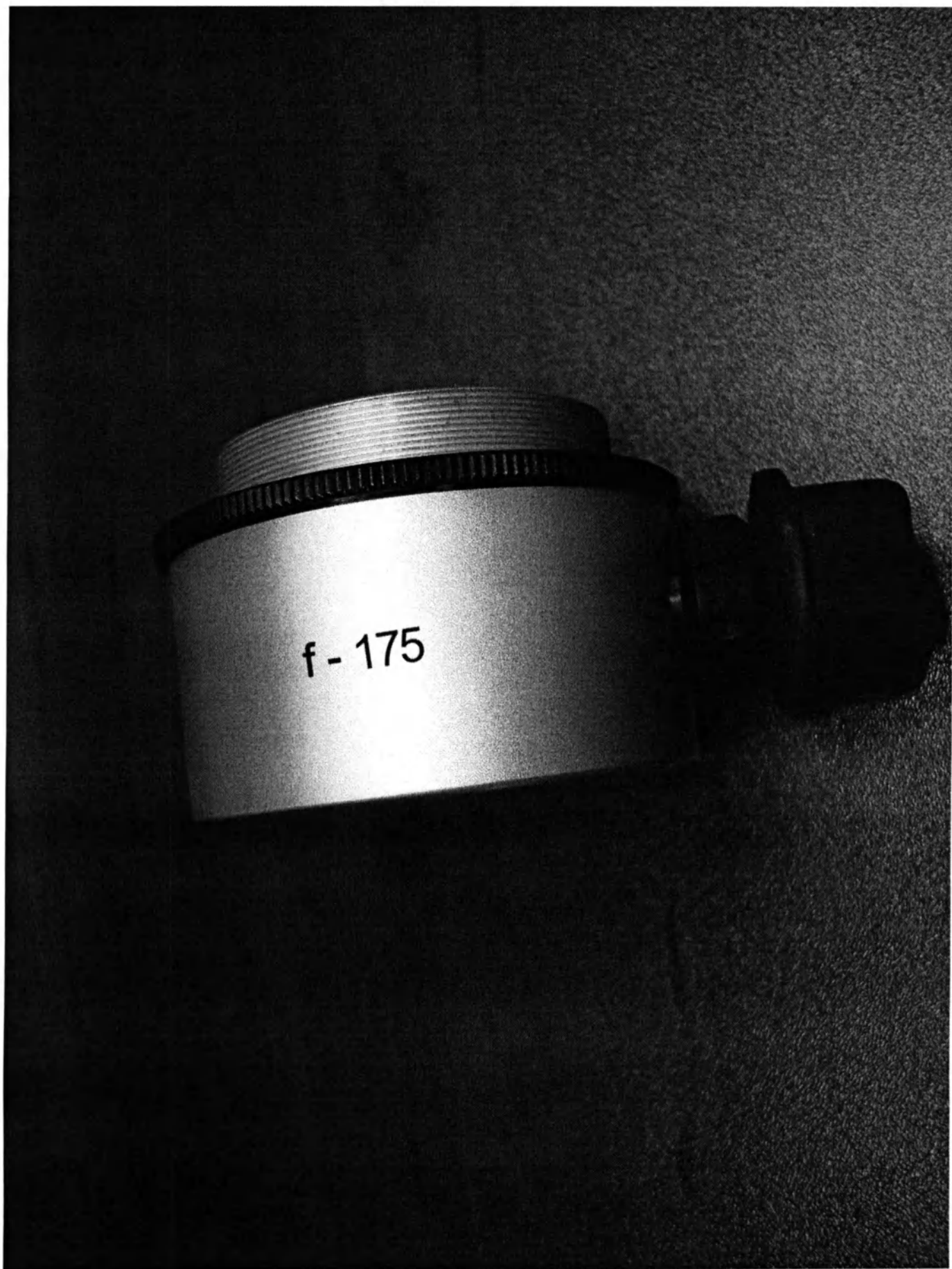
Объектив f=175 мм с механизмом фокусировки со стерилизуемым колпачком
