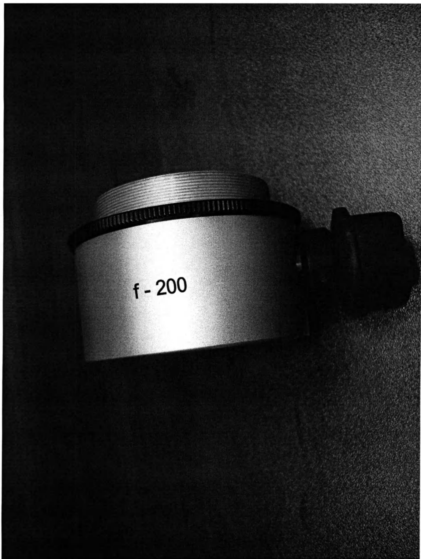
Объектив f=200 мм с механизмом фокусировки со стерилизуемым колпачком
