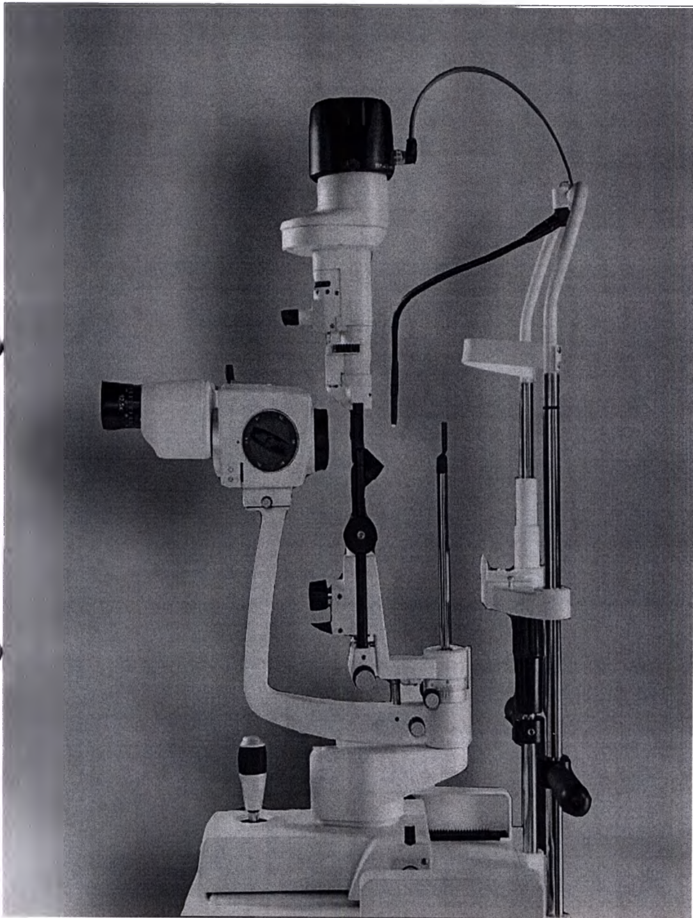
Лампа щелевая eVO 450
