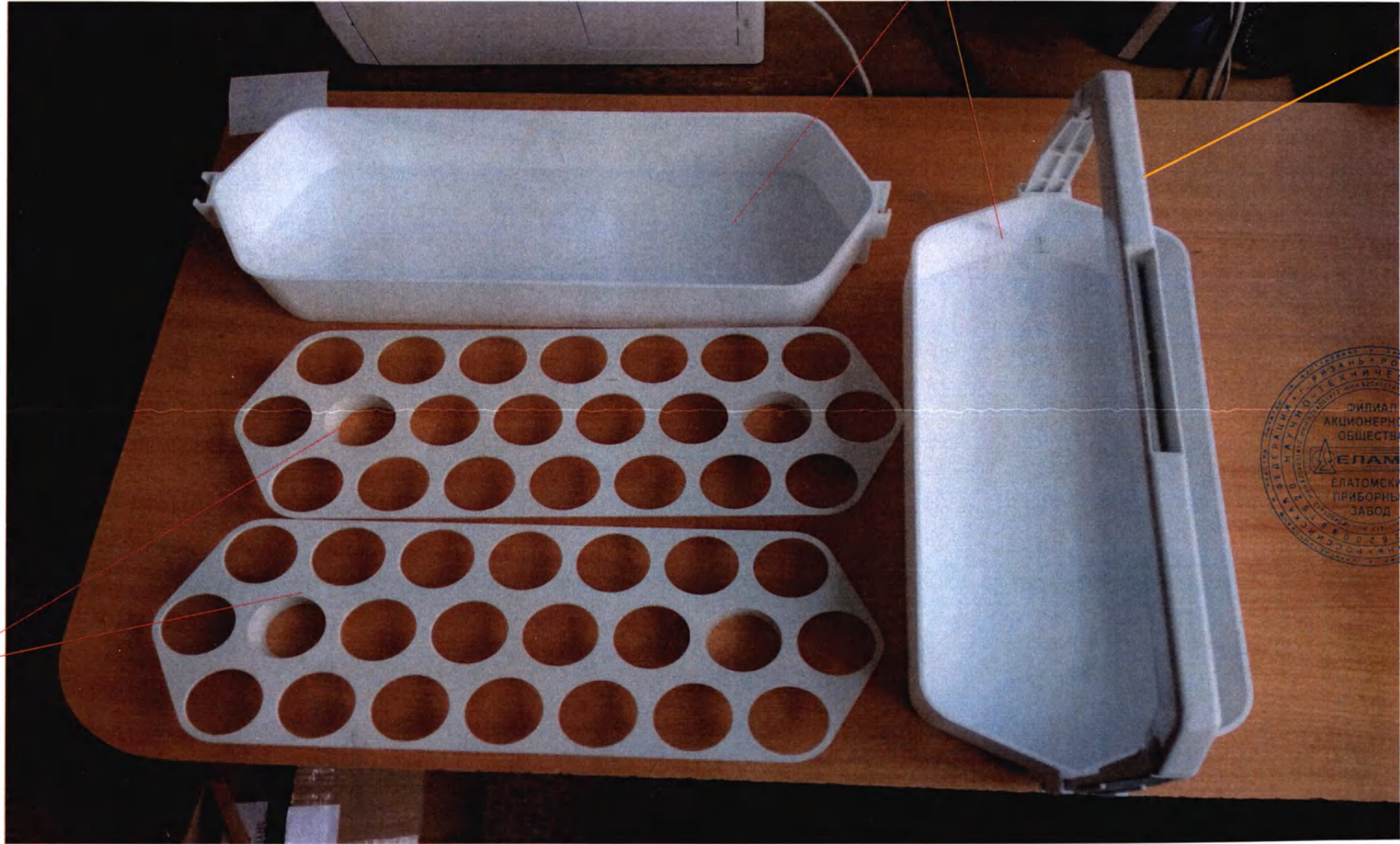
Медицинское изделие «Контейнер для переноса баночек для анализов КПБ-01» по ГИКС.942849.103ТУ в разложенном виде: 1- ложементы; 2 - корпус; 3 – ручка.
