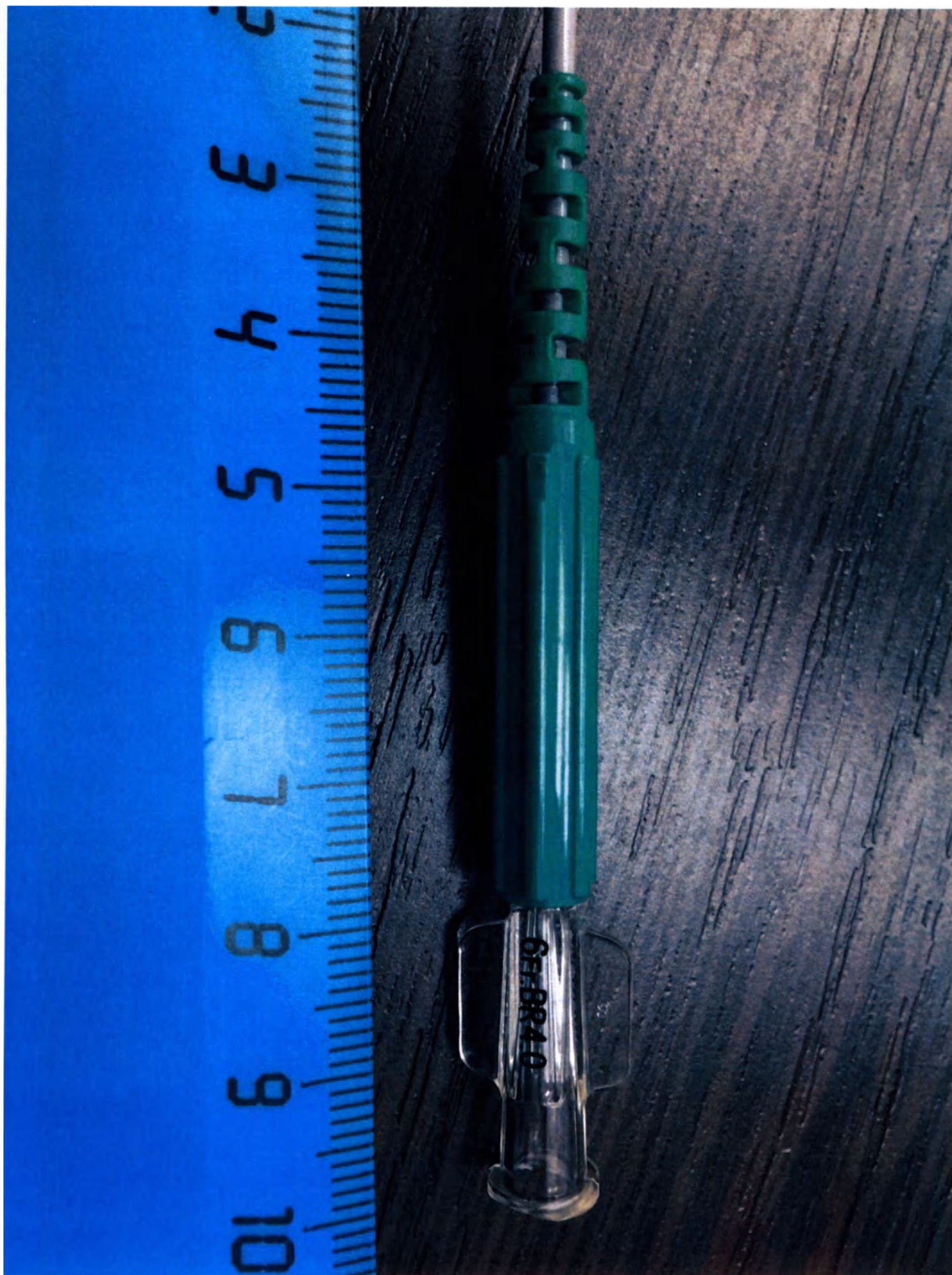
Катетер проводниковый Heartrail II, противозагибочный протектер 6 Fr :
