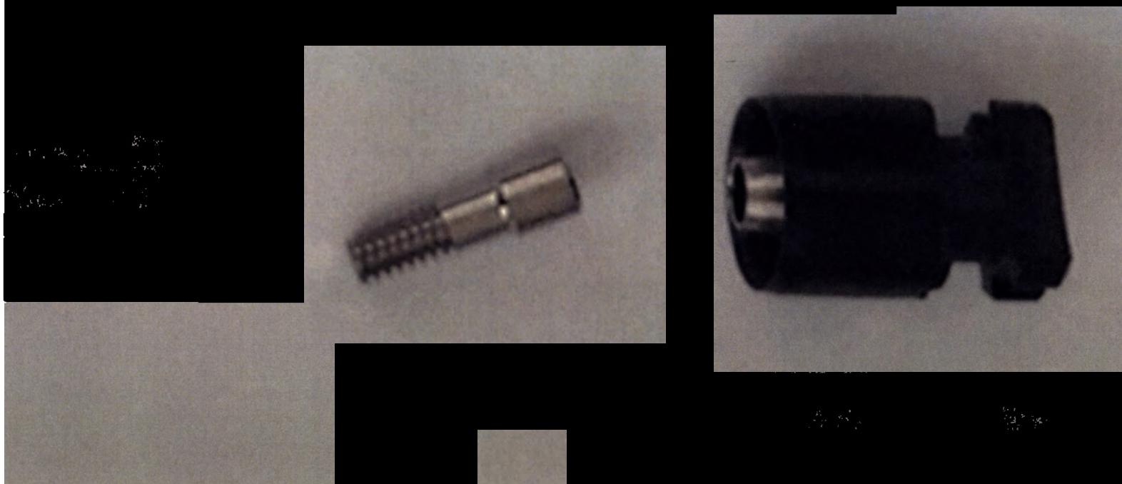
Рис. 8. Колпачок выжигаемый (с винтовой фиксацией) в наборе (колпачок и винт)
