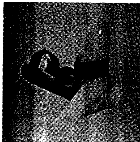
Рисунок 4 Тугор на голеностопный сустав безнагрузочный с деротационным фиксатором ТНО-23
