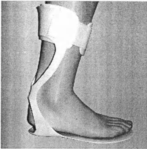
Рисунок 5 Тугор - стоподержатель ТНО-24
