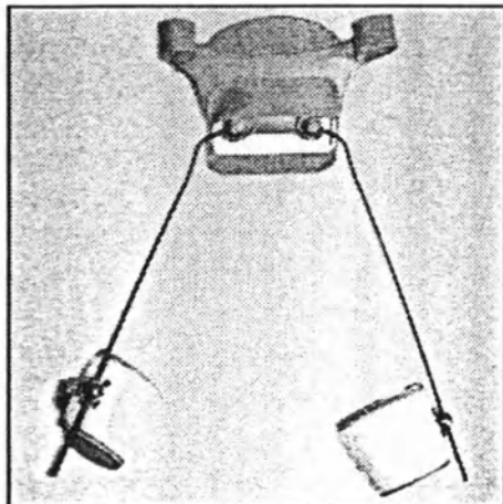
Рисунок 6 - Аппарат для разведения и установки бёдер в заданном положении АН4-12
