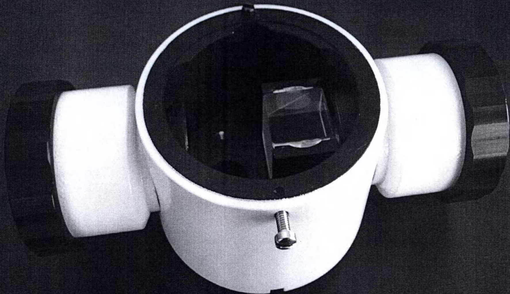
19. Делитель оптического канала 50/50.
