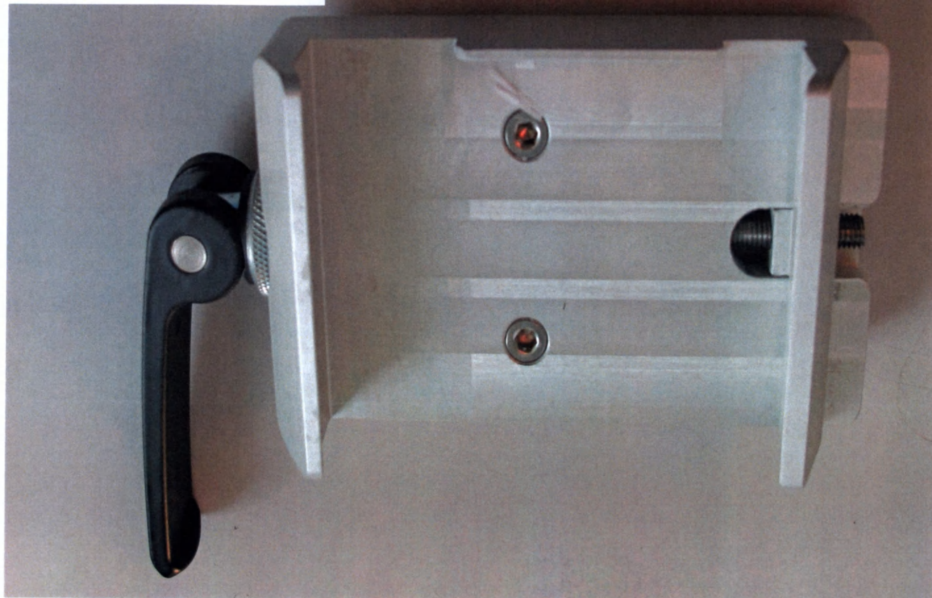
Рис.5. Зажим для мега-кассет
