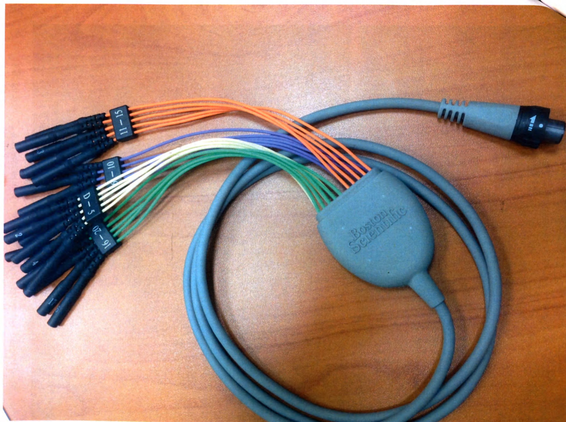
Принадлежность. Кабель для подключения Blazer Dx. (Общий вид)
