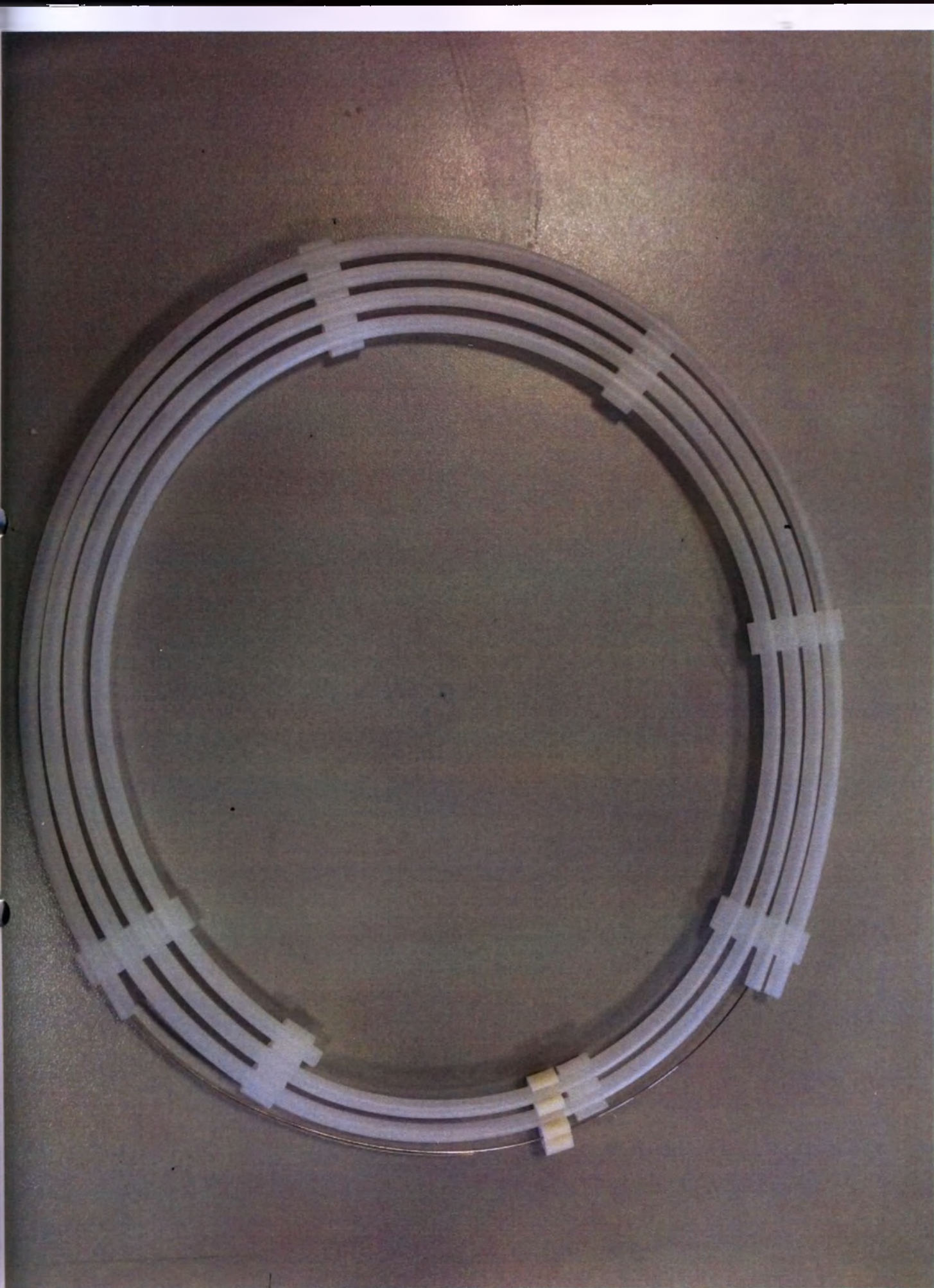
Стент внутрисосудистый Neuroform Atlas, упакованный в диспенсерную катушку с клипсами
