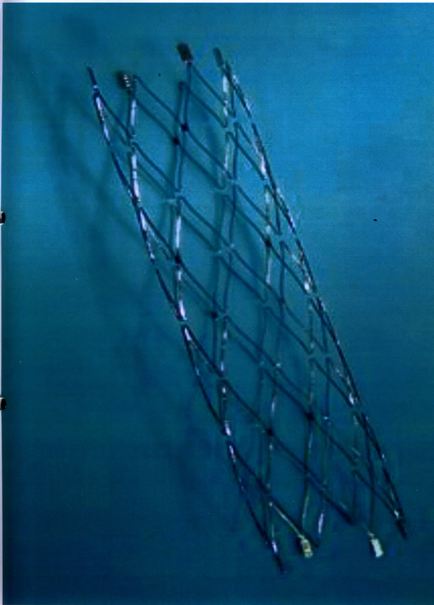
Стент внутрисудистый Neuroform EZ 3. В развернутом виде.
