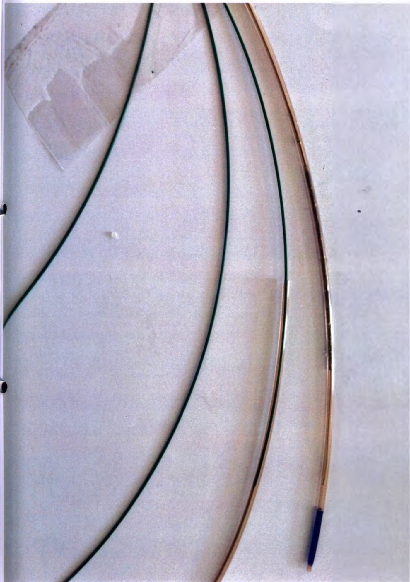
Стент внутрисосудистый Neuroform EZ 3 на системе доставки.
