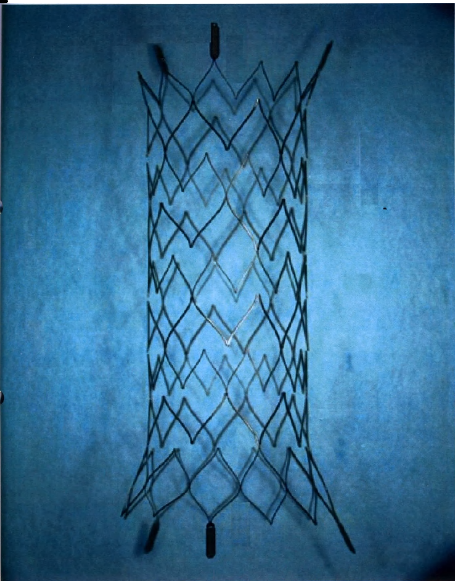
Стент внутрисосудистый Neuroform Atlas в развернутом виде
