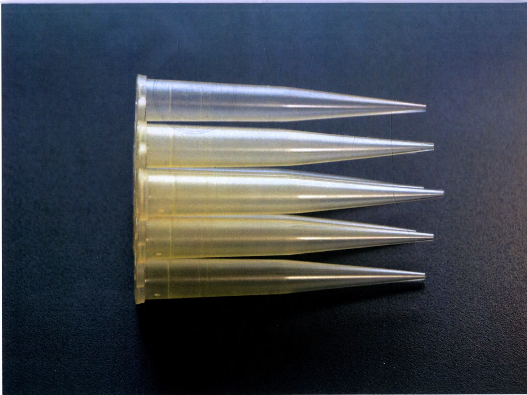
Рис 12. - Наконечник полимерный одноразовый к дозаторам пипеточным НП- «Термо Фишер Сайентифик» для девятиканального дозатора на (200–1000) мкл
