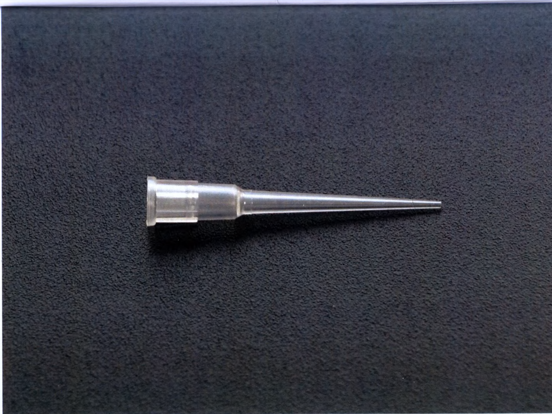
Рис 1. - Наконечник полимерный одноразовый к дозаторам пипеточным НП-«Термо Фишер Сайентифик» для одноканального дозатора на (0,2–10) мкл
