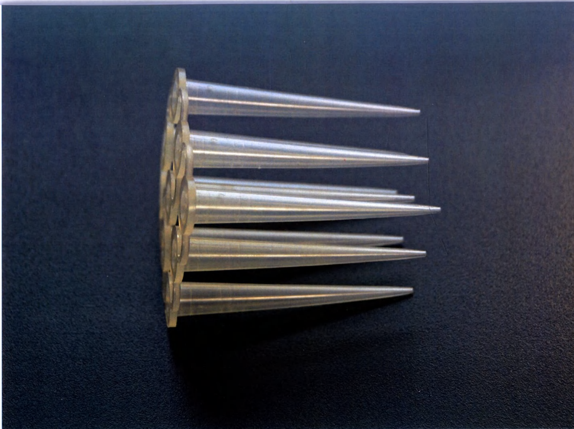
Рис 11. - Наконечник полимерный одноразовый к дозаторам пипеточным НП-«Термо Фишер Сайентифик» для девятиканального дозатора на (5–200) мкл
