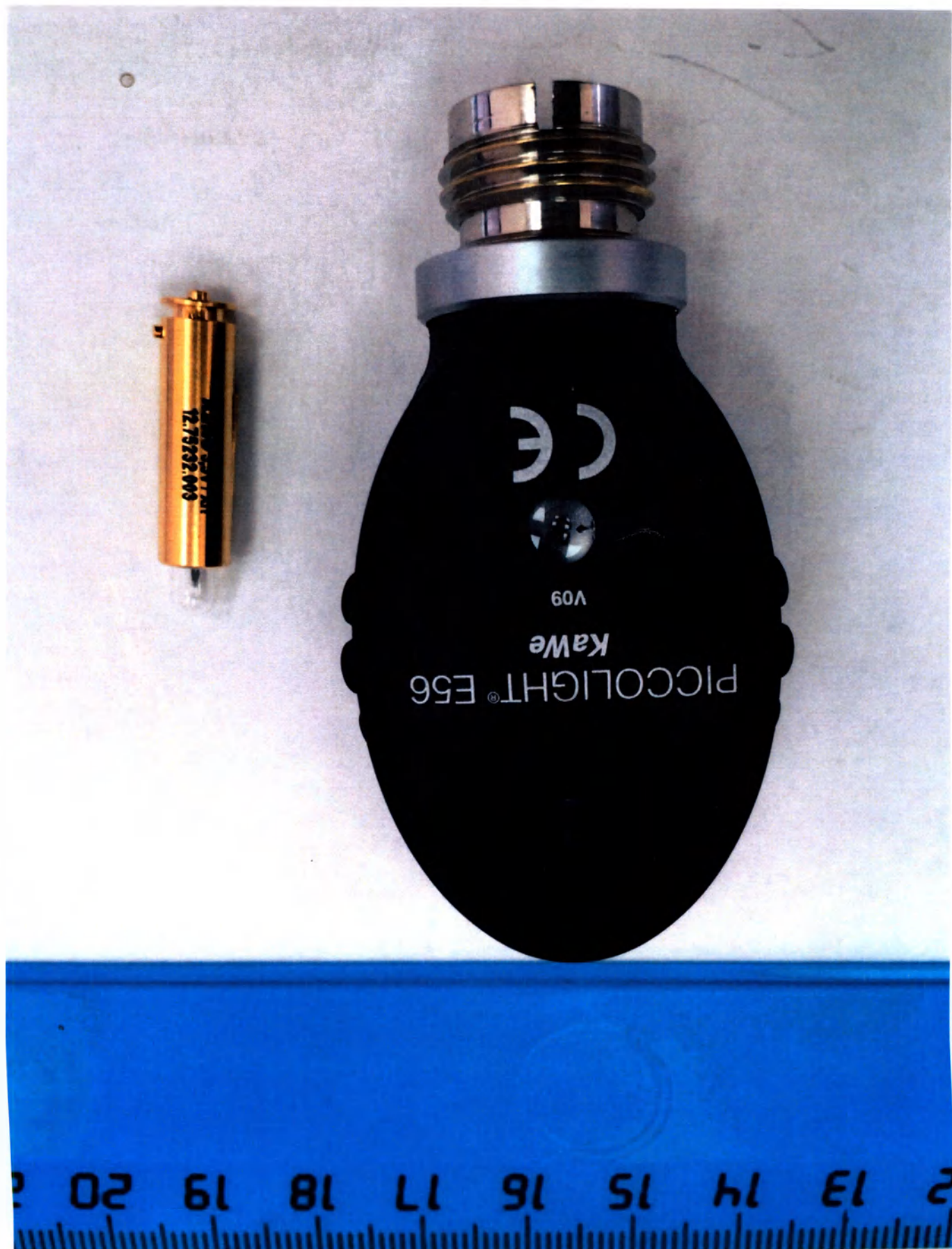
Головка офтальмоскопа Piccolight E56 с источником света ксенон-галогенной лампой (01.87561.021)
