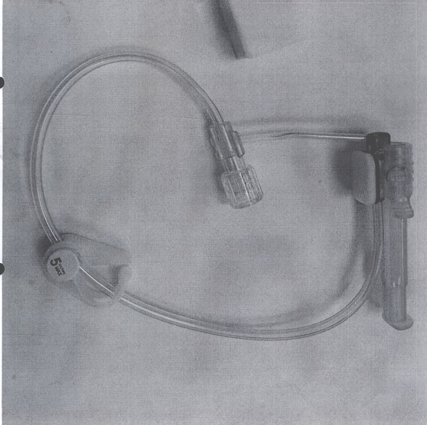
3. Безопасные иглы Губера «ППС Флоу+» (PPS Flow+) без латерального участка инъекции, размер 19G×15 мм.
