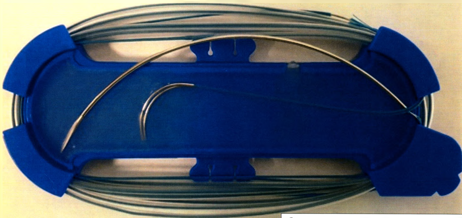
Электрод для временной кардиостимуляции, модель MYWIRE 34
