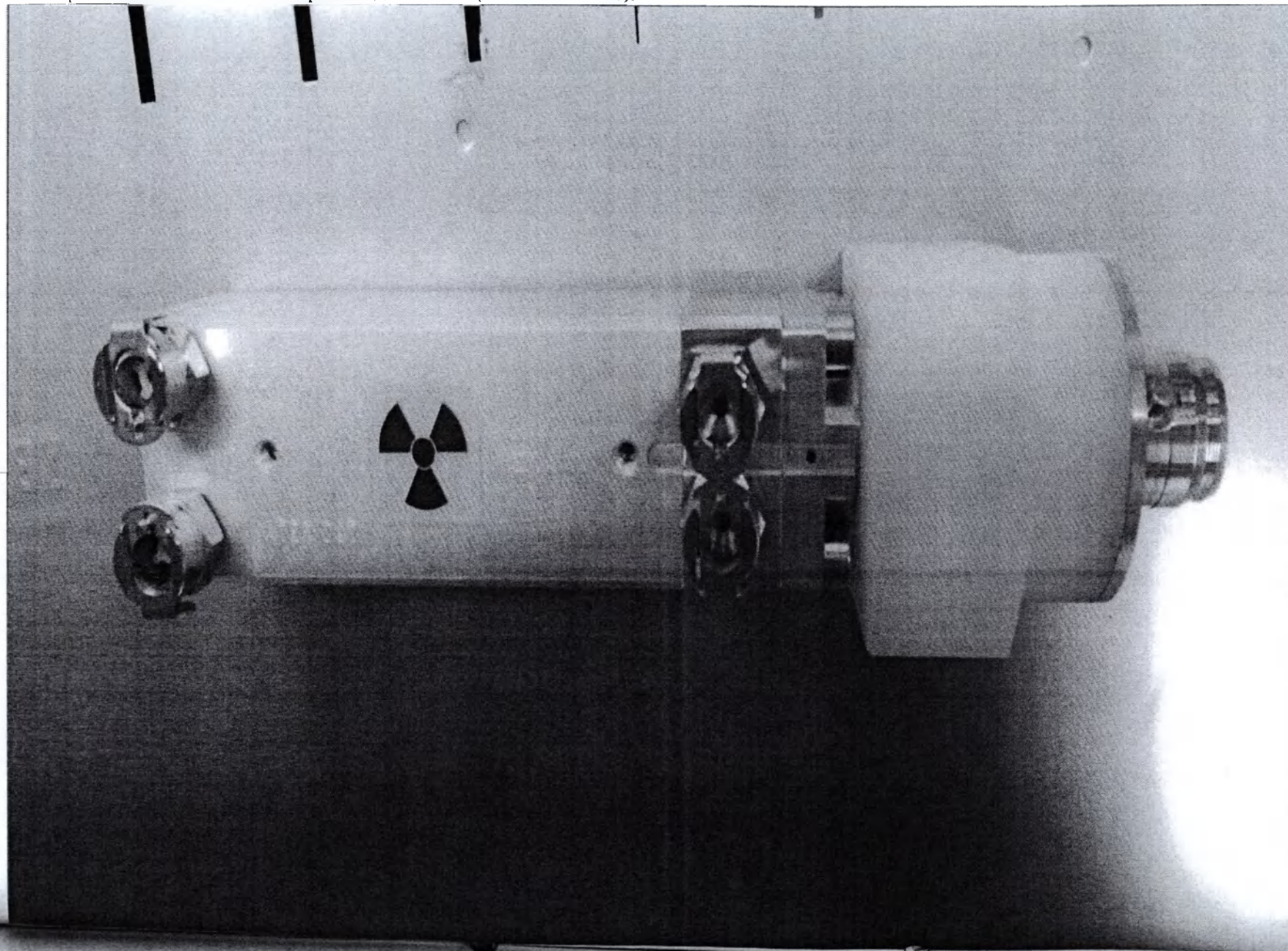
8. Устройство мишенное для производства ИС (не более 8 шт.).
