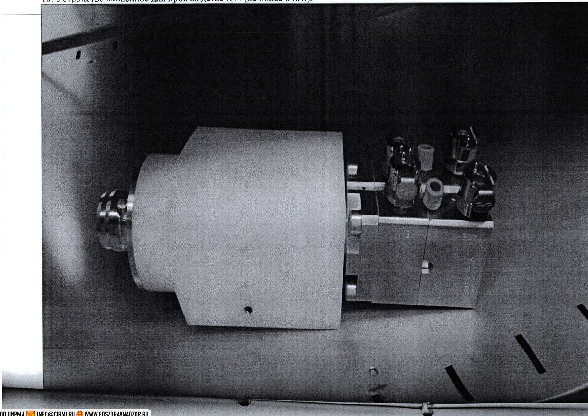
10. Устройство мишенное для производства 13N (не более 8 шт.).
