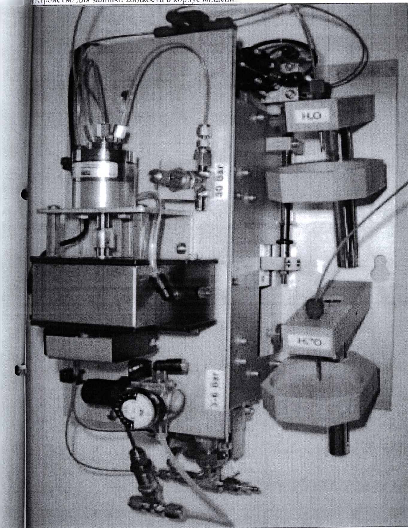
Устройство для заливки жидкости в корпус мишени
