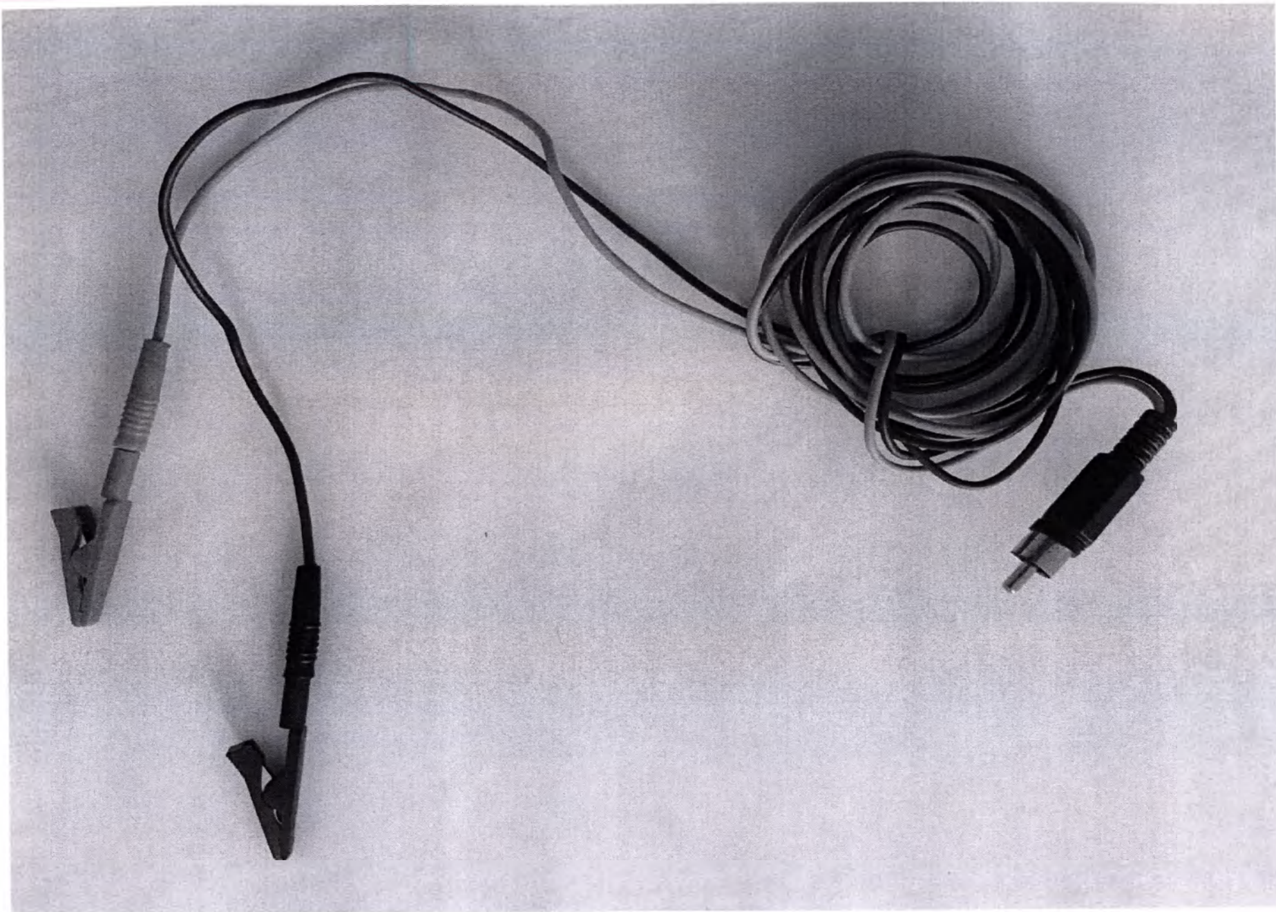
Кабель подключения электродов для низкочастотных электротерапевтических процедур RCA-К-Ч
