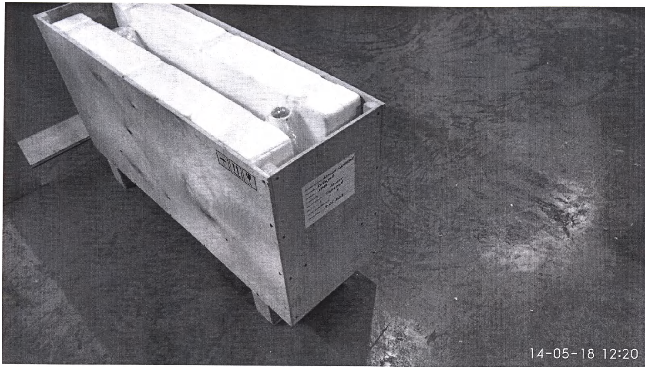
Упаковка двухблочного подвеса Аксима-СД при транспортировке. Вид 2
