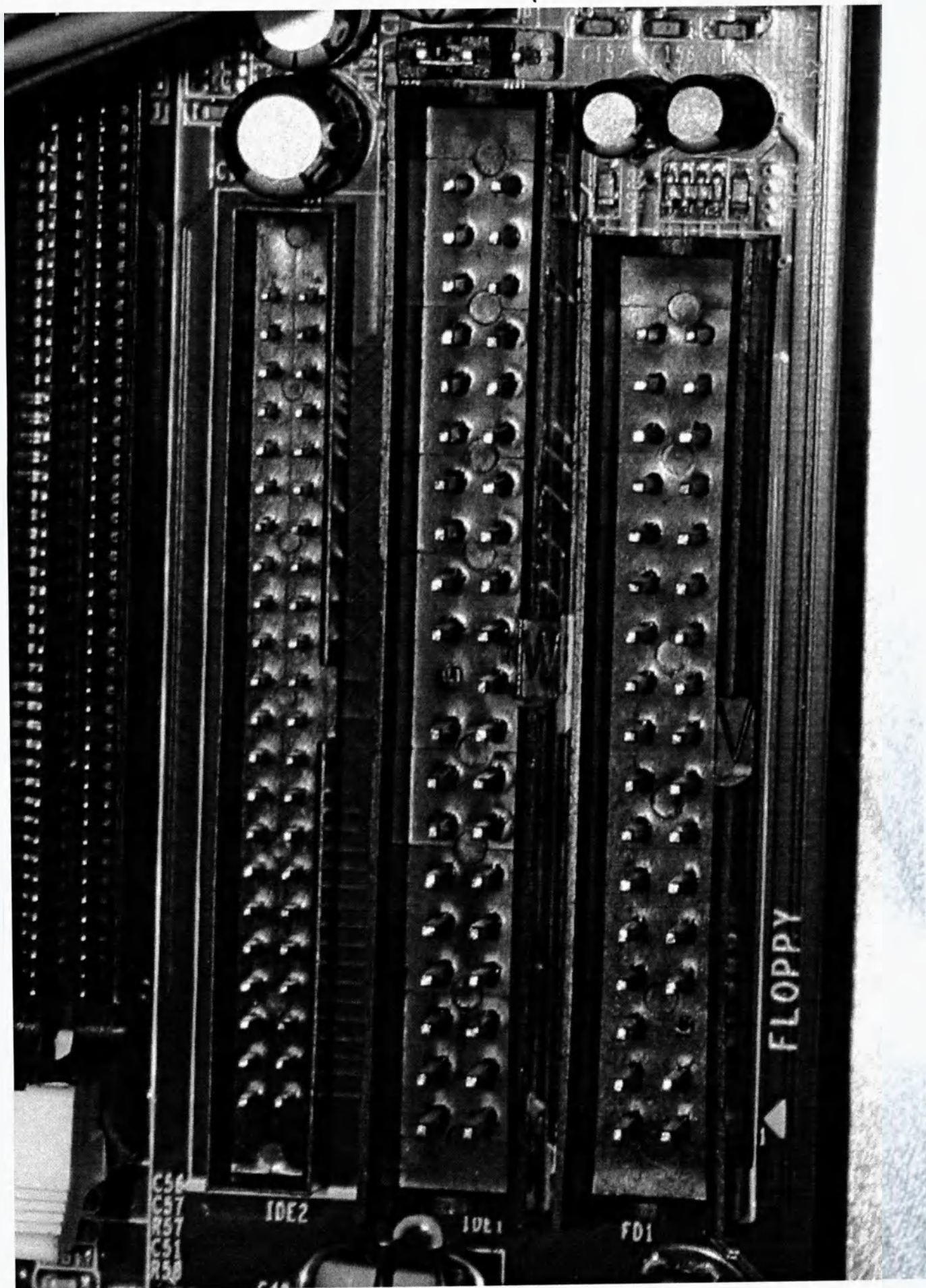
Фото 74 - Контактные элементы из полимеров, металлов и сплавов
