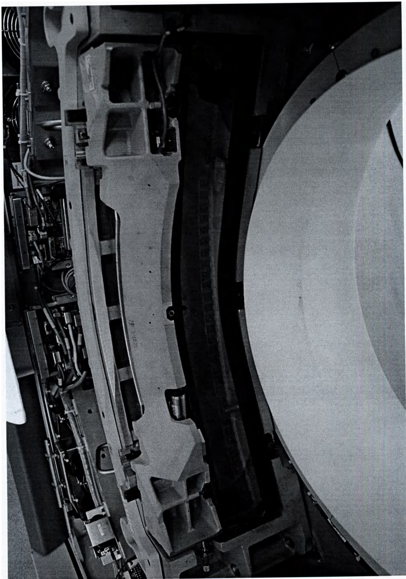
Фото 62 - Детекторы
