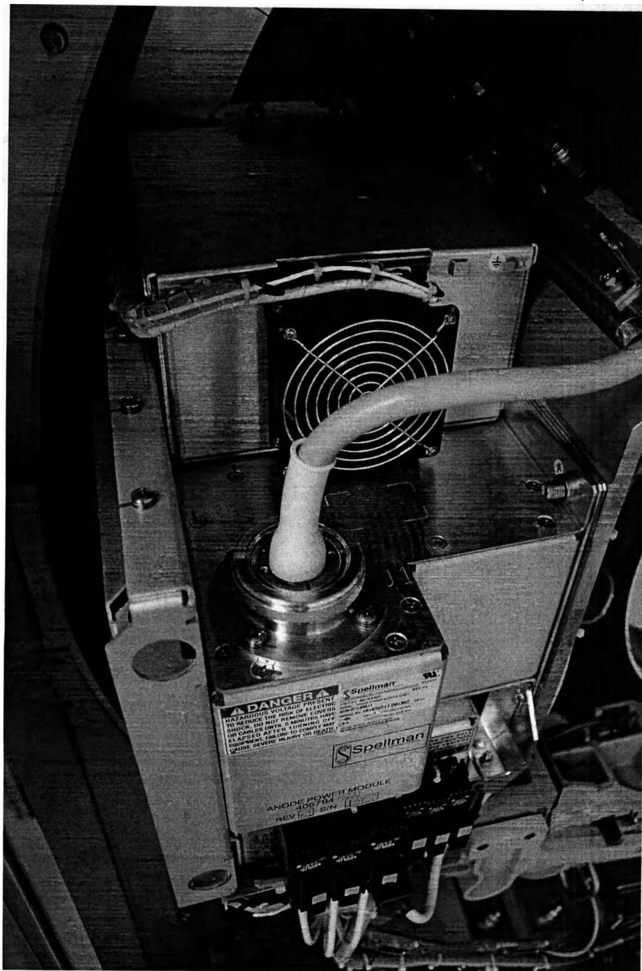
Фото 51 - Высоковольтные генераторы
