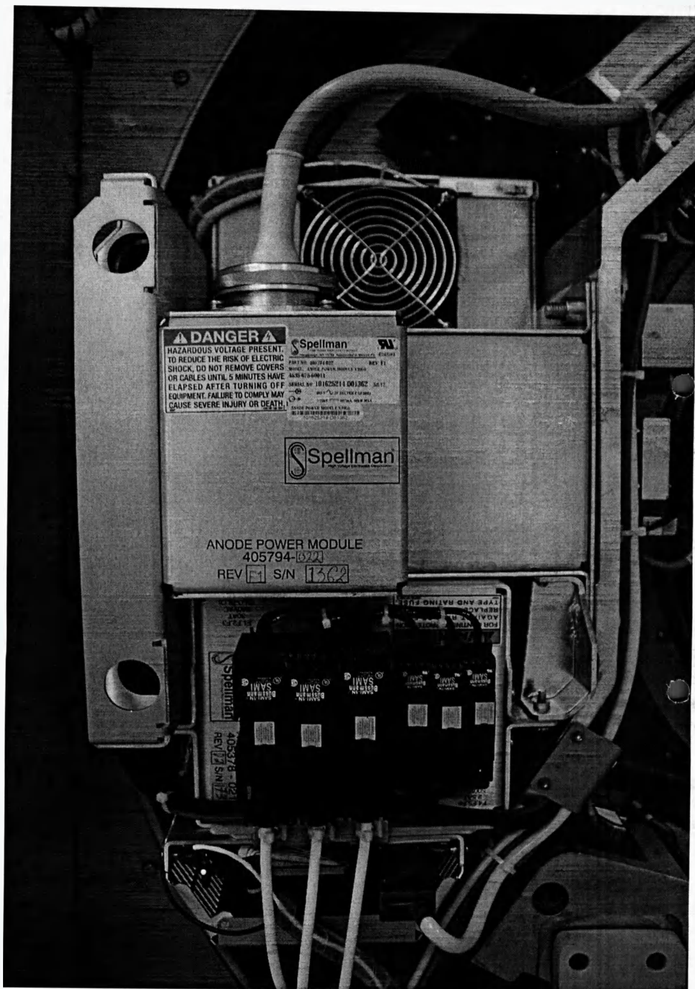
Фото 6 - Рентгеновский высоковольтный генератор
