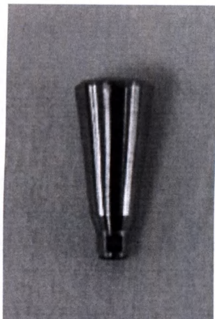
Абатмент фрезеруемый стандартный конический с шестигранником, диаметр 4,80 мм (М), длина 13,1 мм, высота 10 мм
