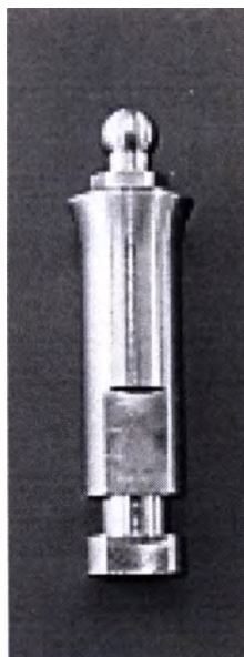
Аналог цельного шаровидного абатмента (аттачмента), диаметр 4,80 мм (М), длина 17,93 мм
