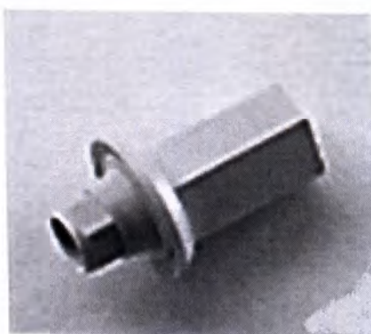
Трансфер сканируемый пластиковый, диаметр 5,80 мм (W), длина 9,75 мм
