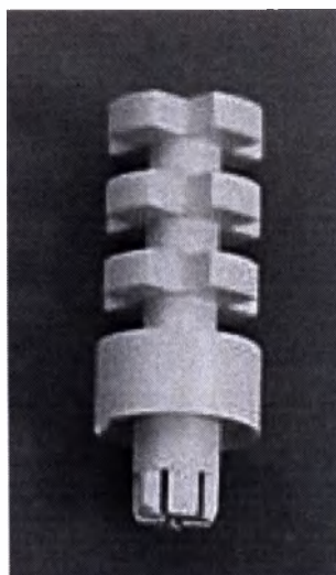
Трансфер Pull-up, диаметр 4,80 мм (М), длина 12,35 мм
