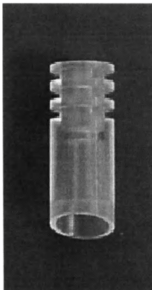
Цилиндр выжигаемый для постоянных угловых 20 град. абатментов, диаметр 4,80 мм (М), длина 12,7 мм
