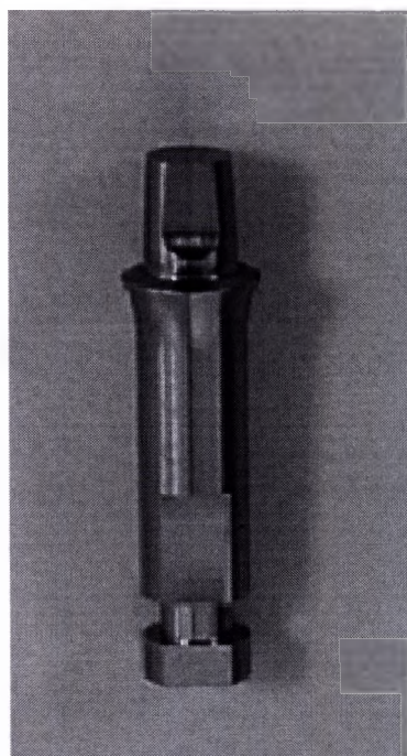
Аналог прямого цельного абатмента диаметр 4,80 мм (М), длина 18,6 мм, высота 4 мм
