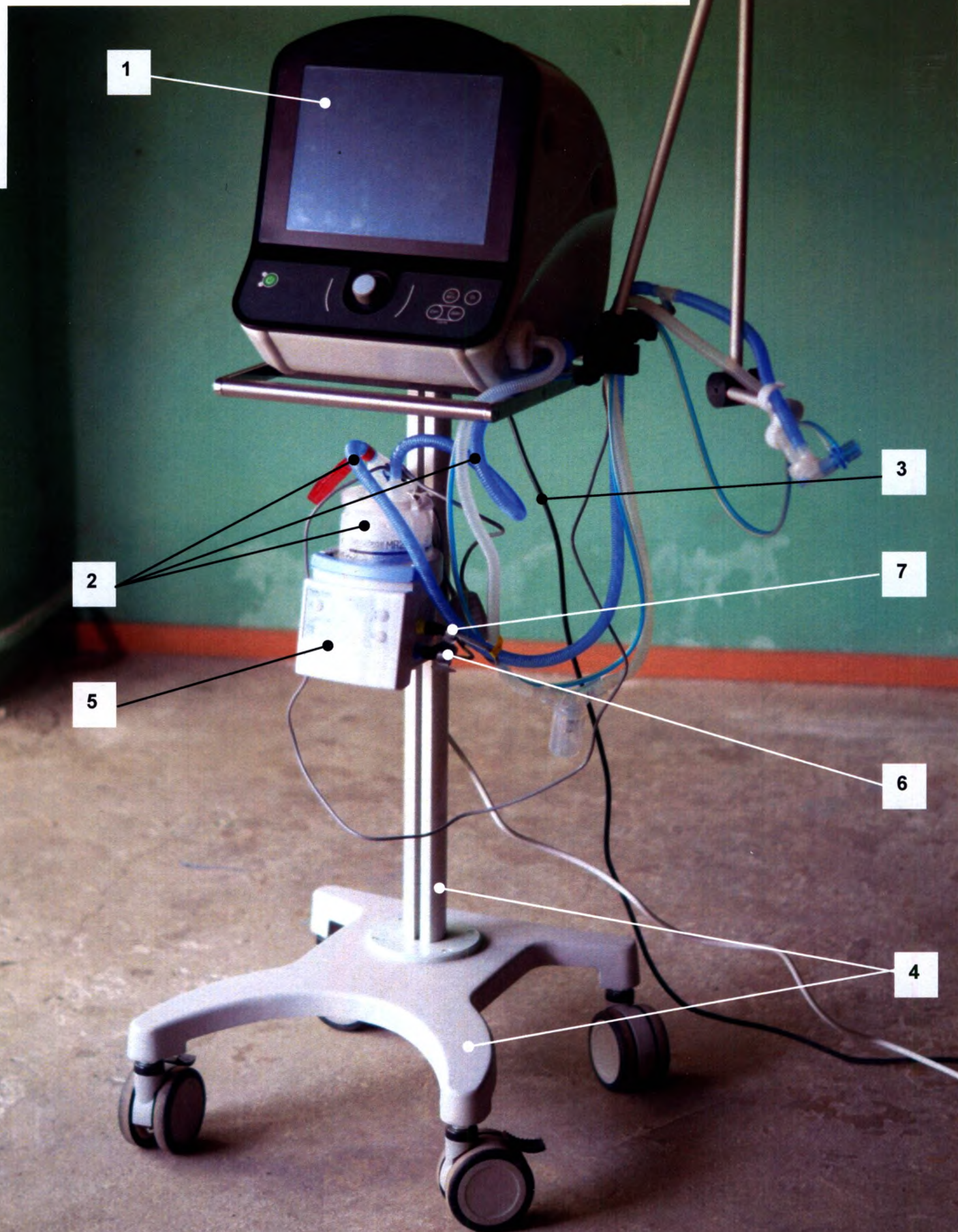
Рисунок 1 - Аппарат искусственной вентиляции лёгких неонатально-педиатрический «Прана» дА 2.931.018. Общий вид, где: 1 - блок вентиляции дА 2.931.019; 2 - неонатальный дыхательный контур опорного потока RT225 с камерой MR290; 3 - шнур питания; 4 - стойка дА 4.110.005; 5 - увлажнитель дыхательных смесей MR850; 6 - температурный датчик для увлажнителя, вариант исполнения 900MR869; 7 - кабель гибкого нагревателя, вариант исполнения 900MR805
