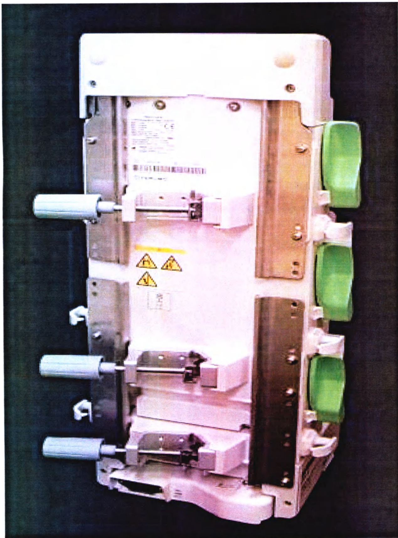
Коммуникационная стойка Terufusion Communication Rack System (вид сзади).
