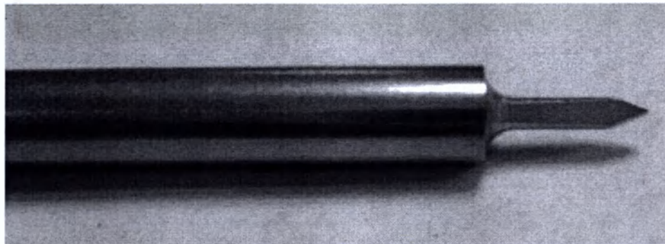
Направитель сверла 1,5мм x 170мм
