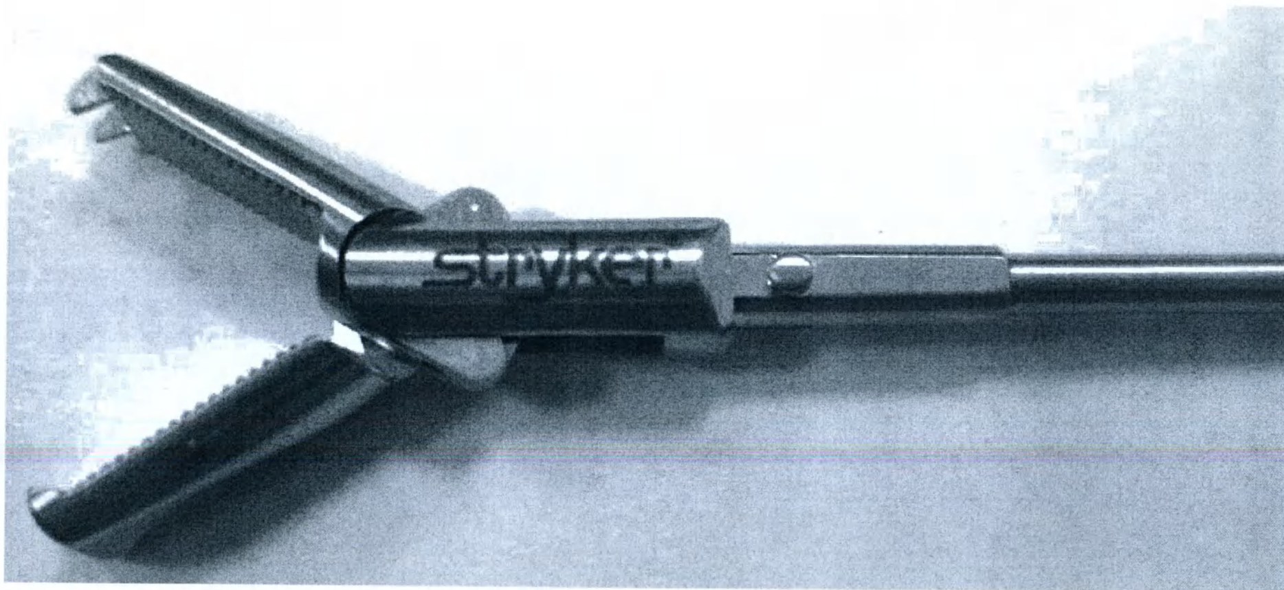
Вставка «граспер» Cobra, диаметр 5 мм, длина 33 см
