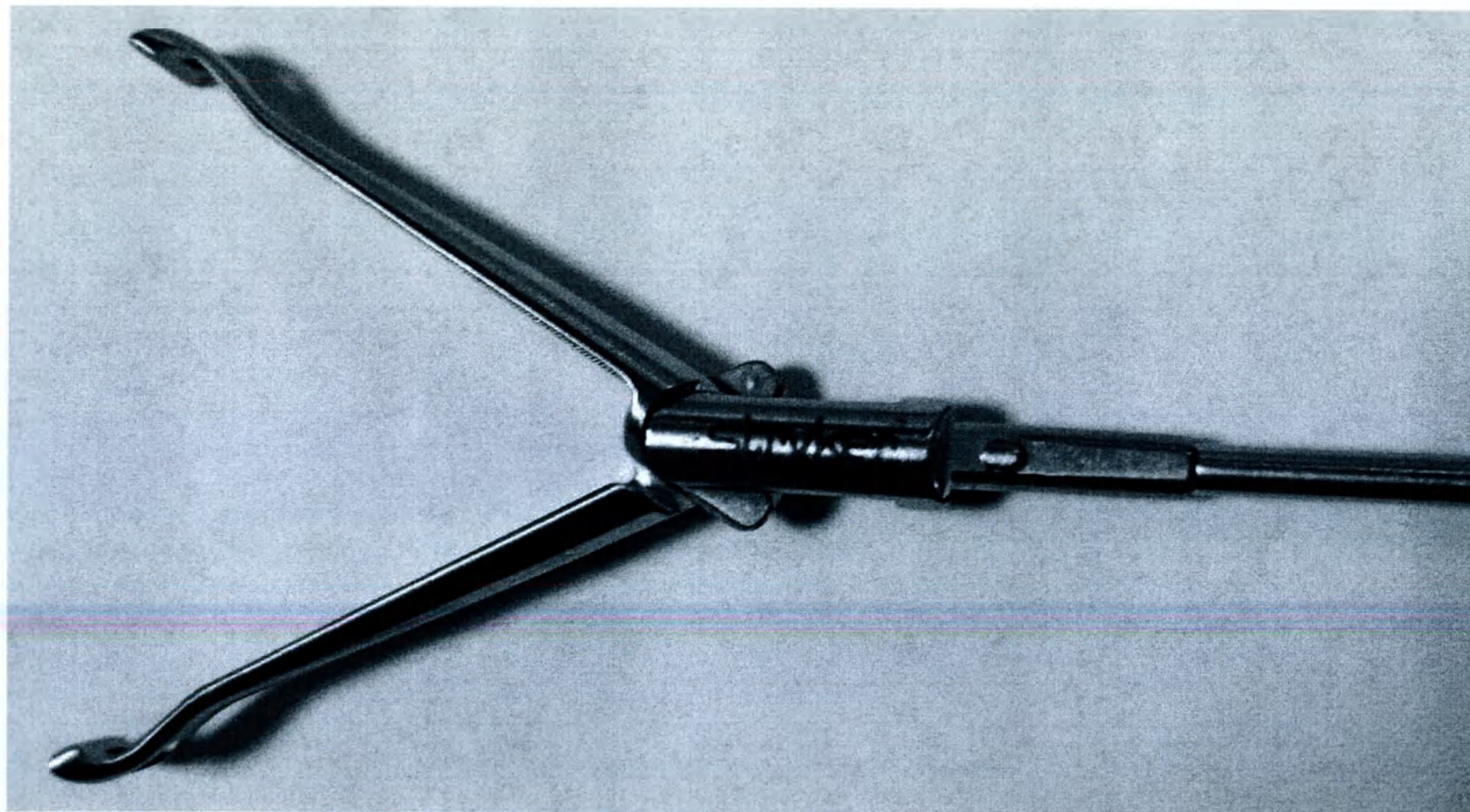
Вставка «граспер» по Бэбкок, диаметр 5 мм, длина 45см
