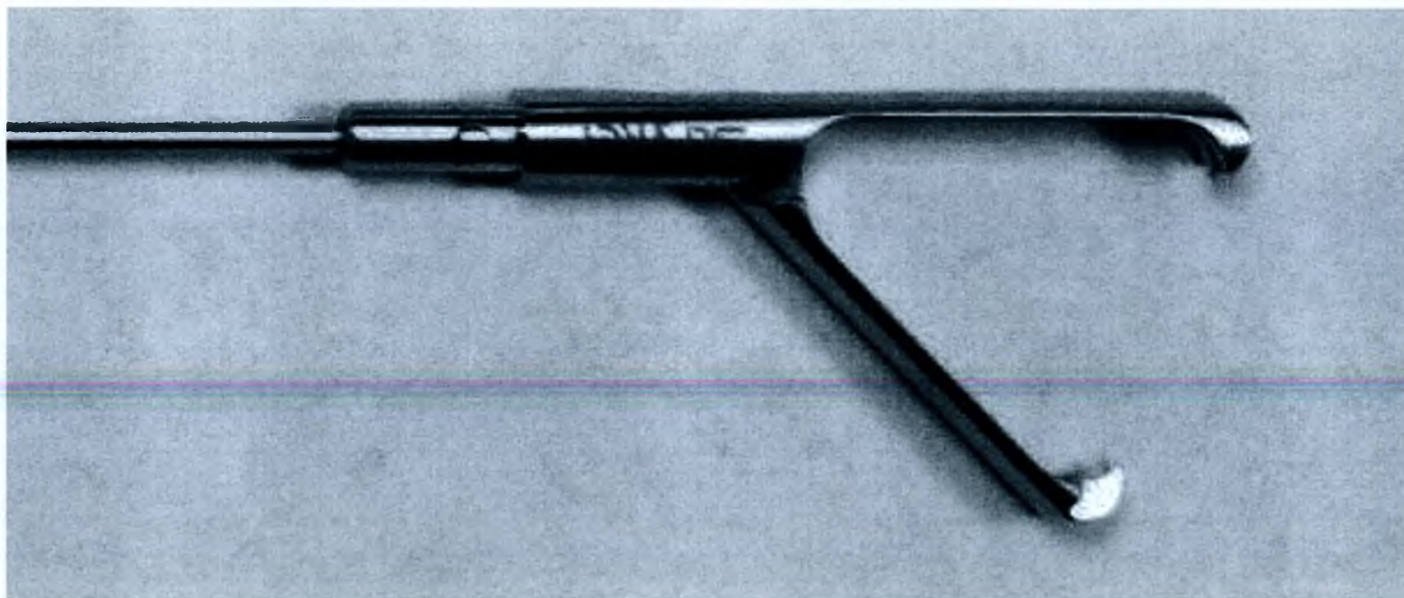
Вставка «граспер» когтеобразная, диаметр 10 мм, длина 33см, с одной подвижной branшей
