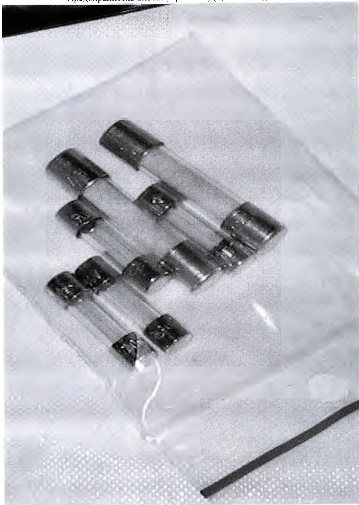
Предохранитель 2х10ат (с резьбой) (6,3 x 32 мм), 2 шт.
