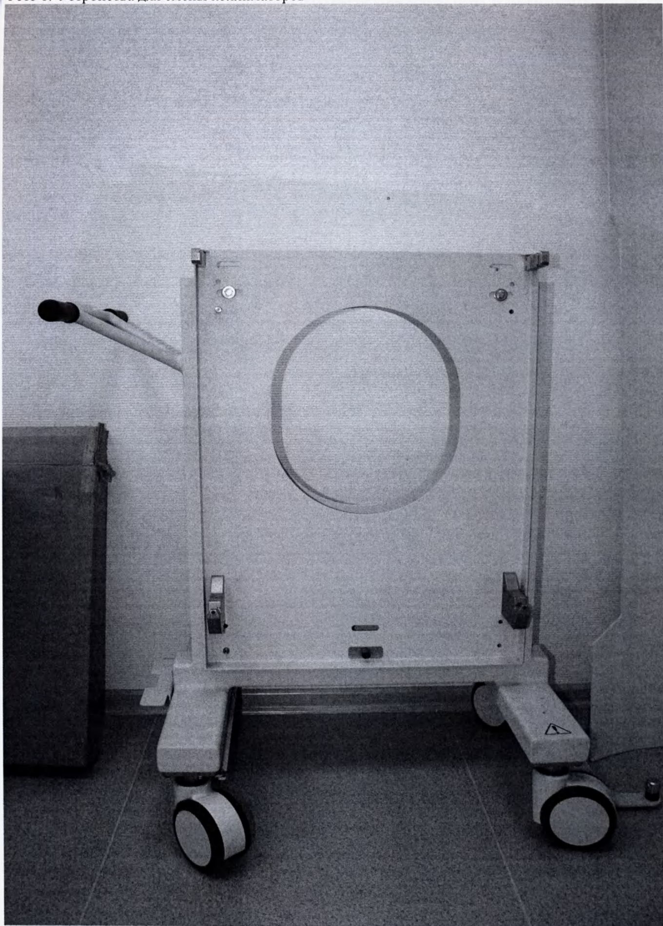
Фото 8. Устройства для смены коллиматоров
