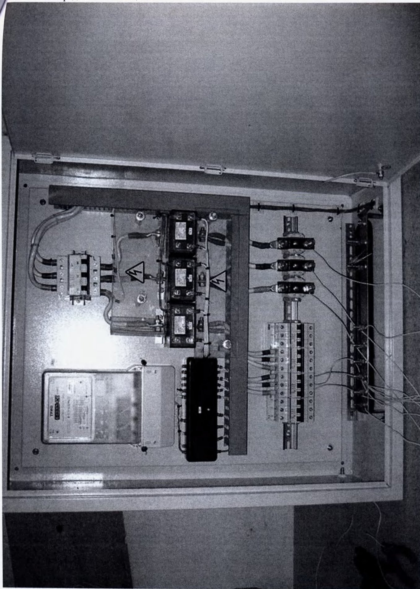
фото 45. Распределительные щиты
