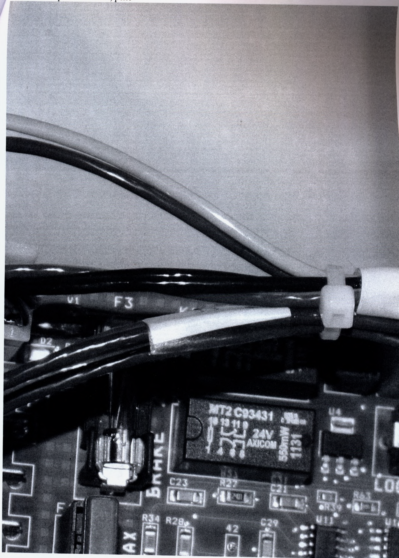
Фото 58. Переключатели, реле
