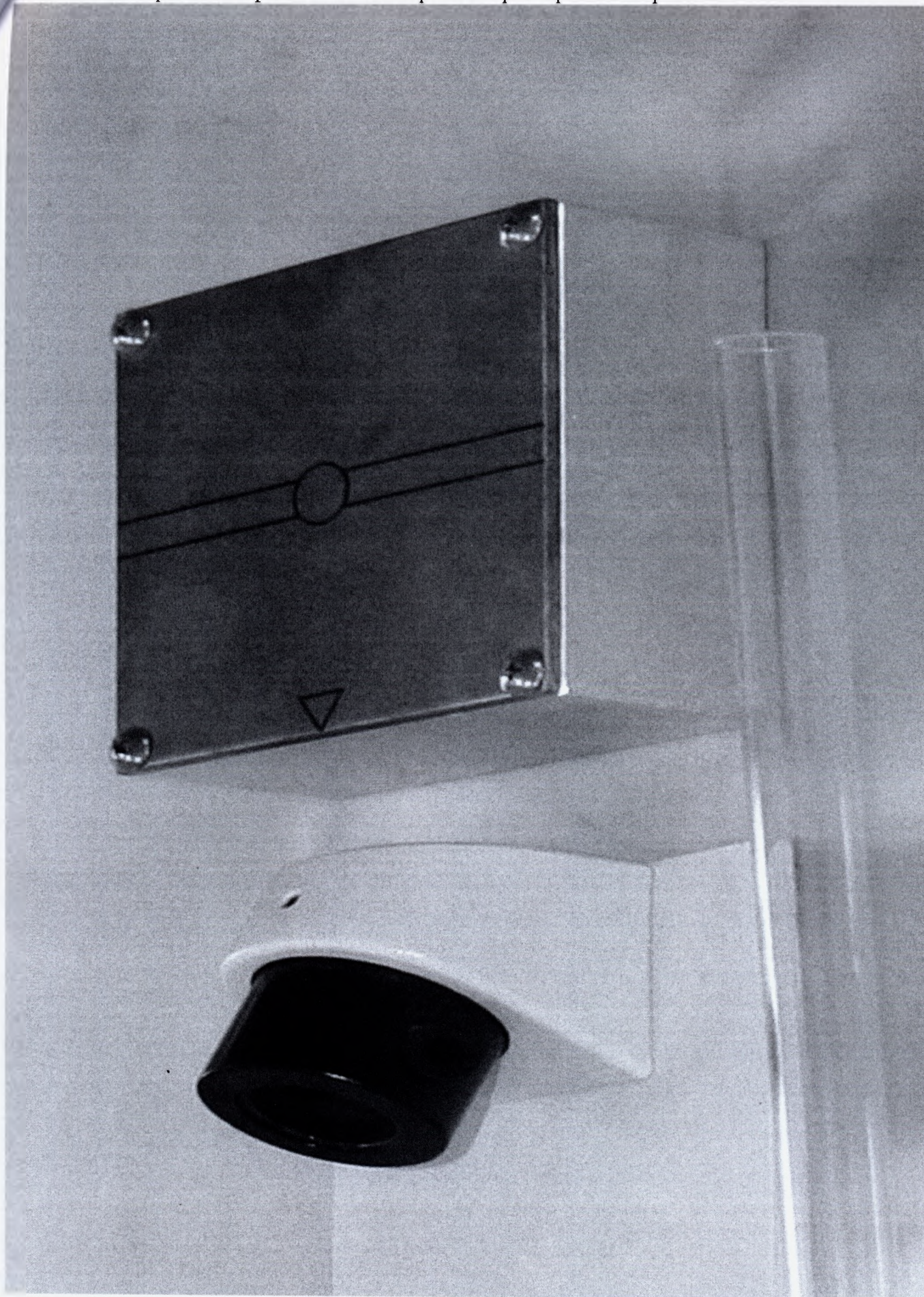
Фото 12. Калибровочные фантомы для настройки параметров и контроля качества
