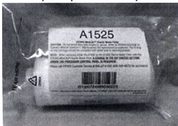
24. Фильтр для производства стерильной воды, с удлиненным сроком службы (A1525).
