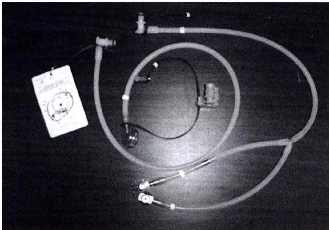
11. Переходник для внутренних каналов эндоскопов Fujinon .
