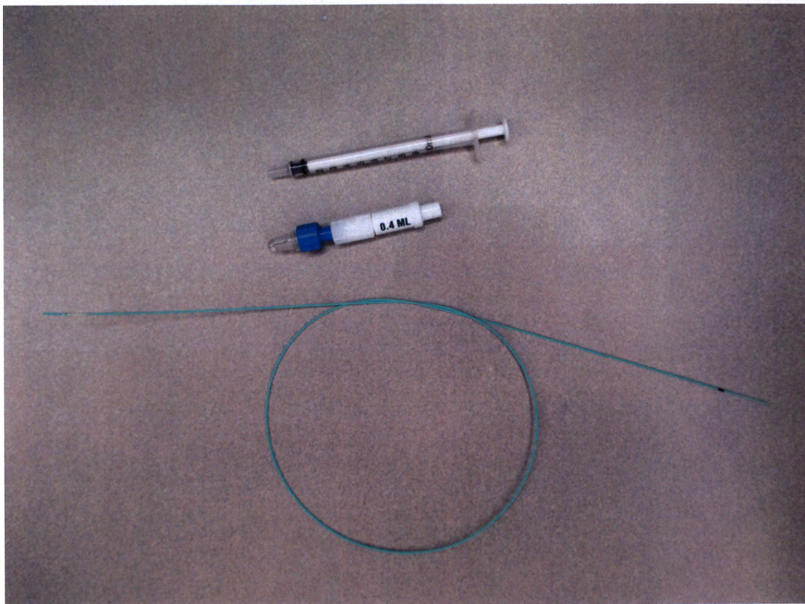
Катетер Ureteroscopy Occlusion Balloon Catheter с адаптером и шприцем, объемом 1 мл (028003)
