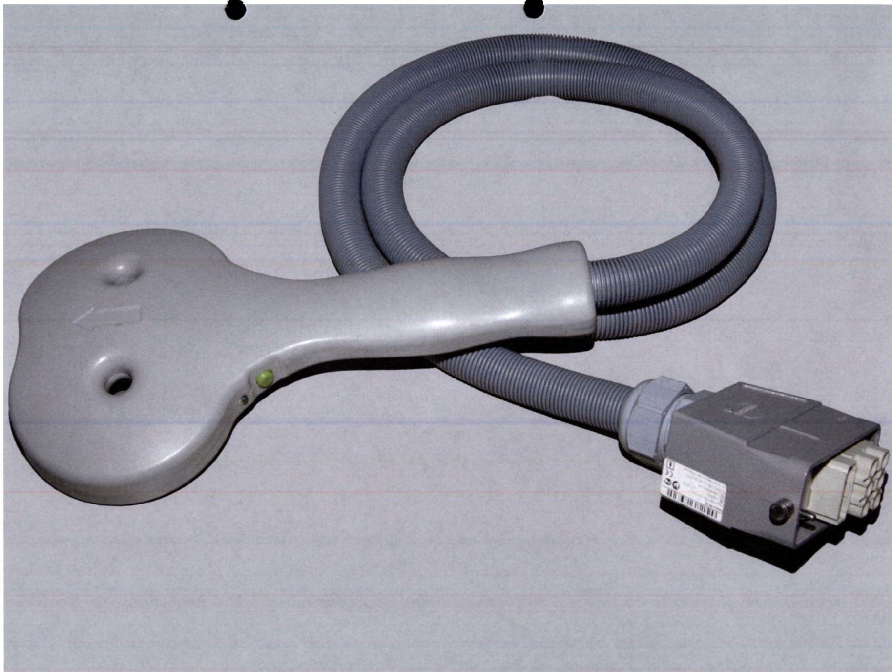
Индуктор двойной угловой 100 мм «ИДУ-02-100»
