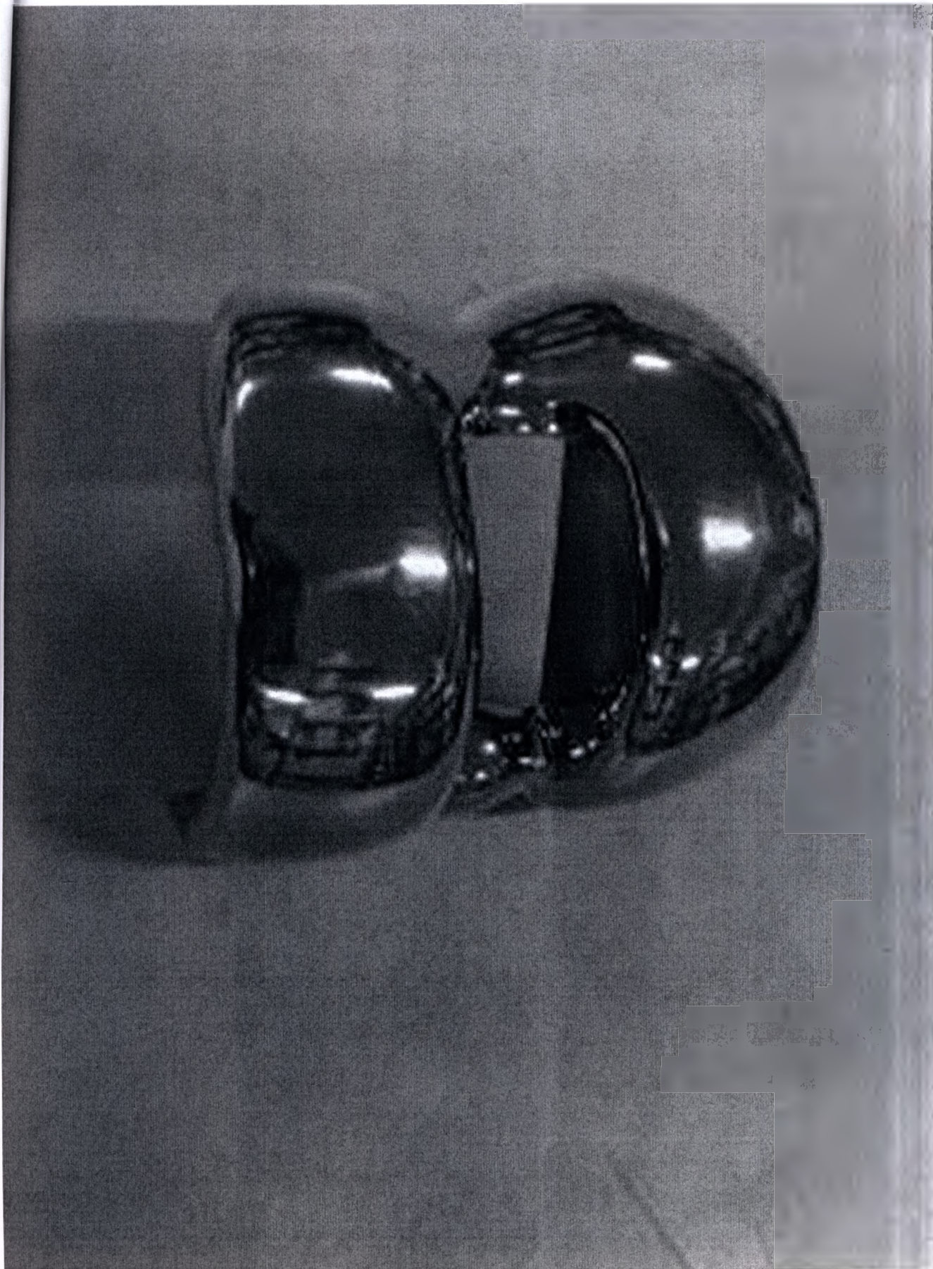
Мышелки бедренной кости с задним стабилизатором с Ti покрытием, левые
