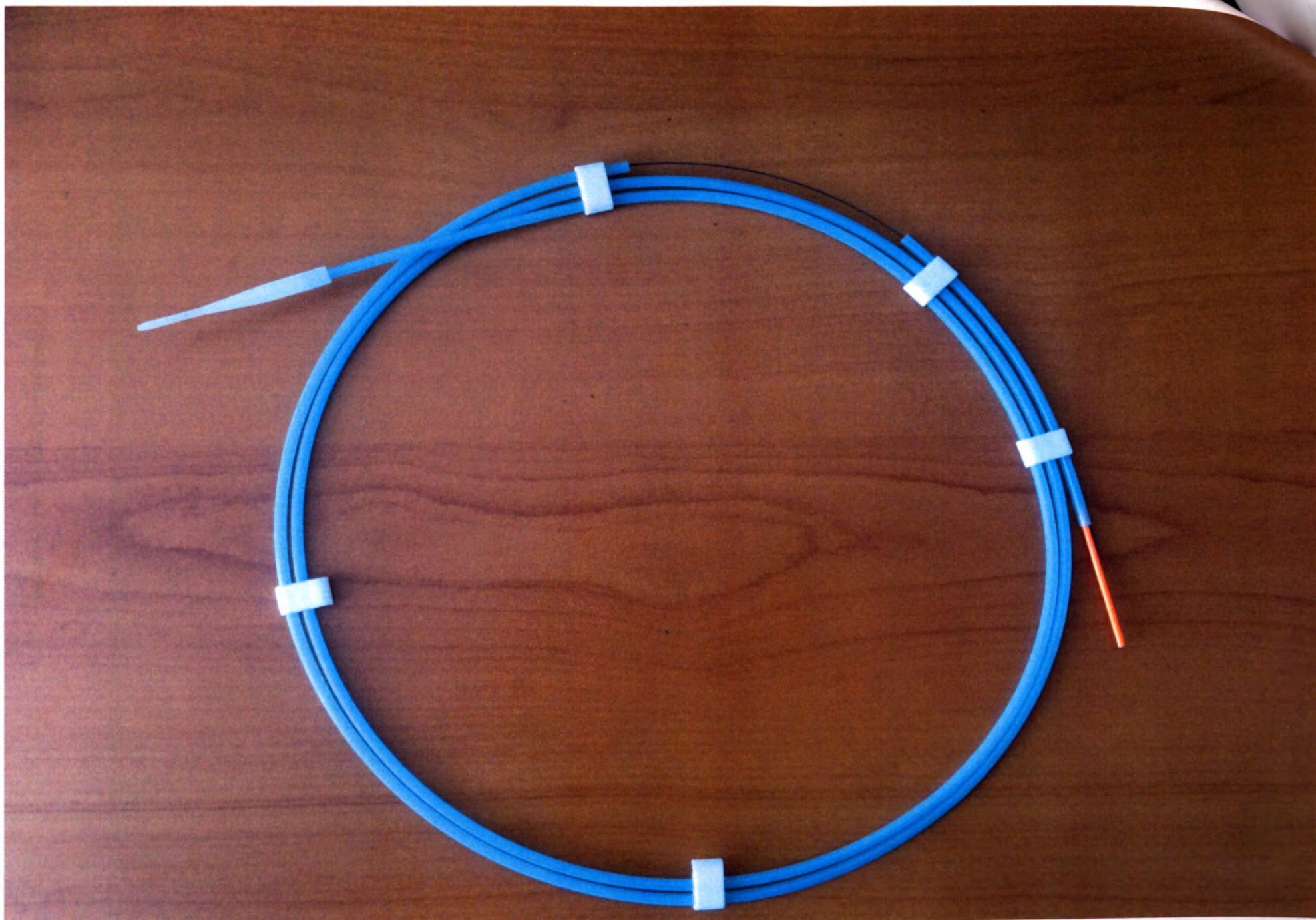
Удлинитель проводника для ЧТКА Runthrough NS Extension Wire: общий вид в держателе
